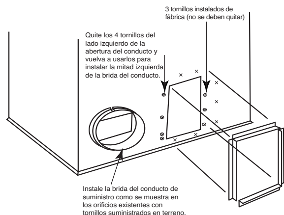
Fig. 3: Instalación de las bridas para los conductos suministradas de fábrica
