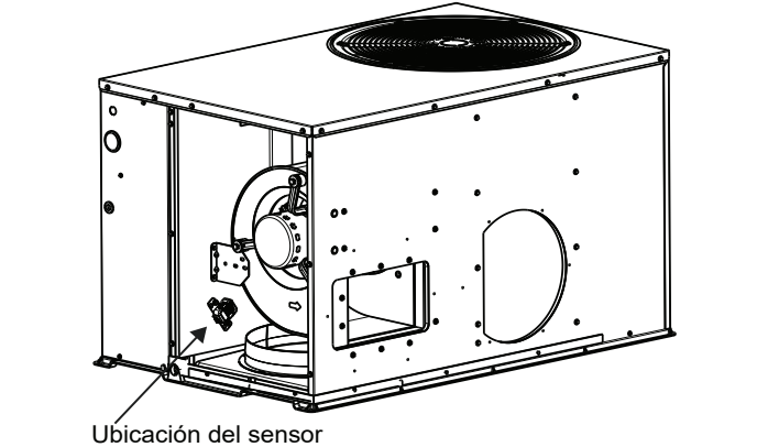
Fig. 13: Ubicación del sensor A240402SP
