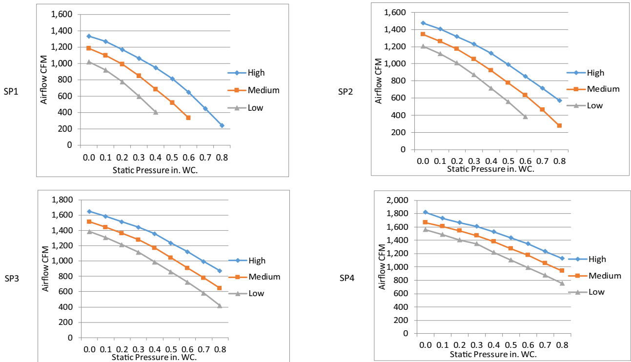
Fig. 10 — Fan Performance - 36K
