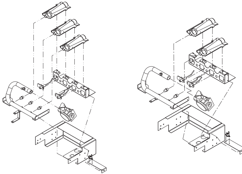
Fig. 15 - Monoport Burner
