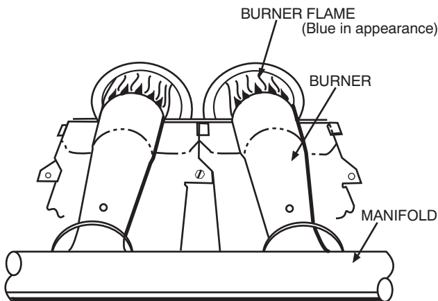
Fig. 6 - Monoport Burner
