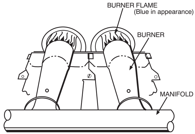
Fig. 15 - Monoport Burner
