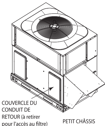
Fig. 3 – Accès au filtre à petit châssis
