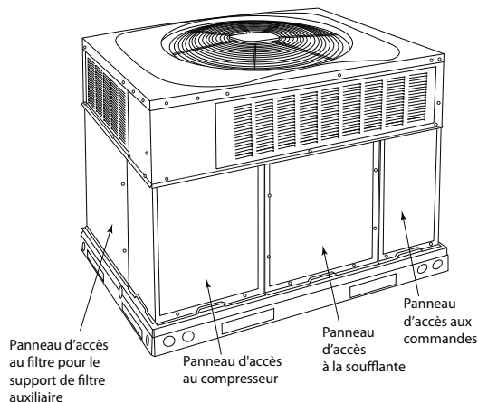
Fig. 2 – Panneau d'accès de support accessoire de filtre
