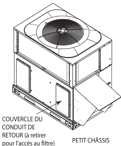
Fig. 3 – Accès au filtre à petit châssis
