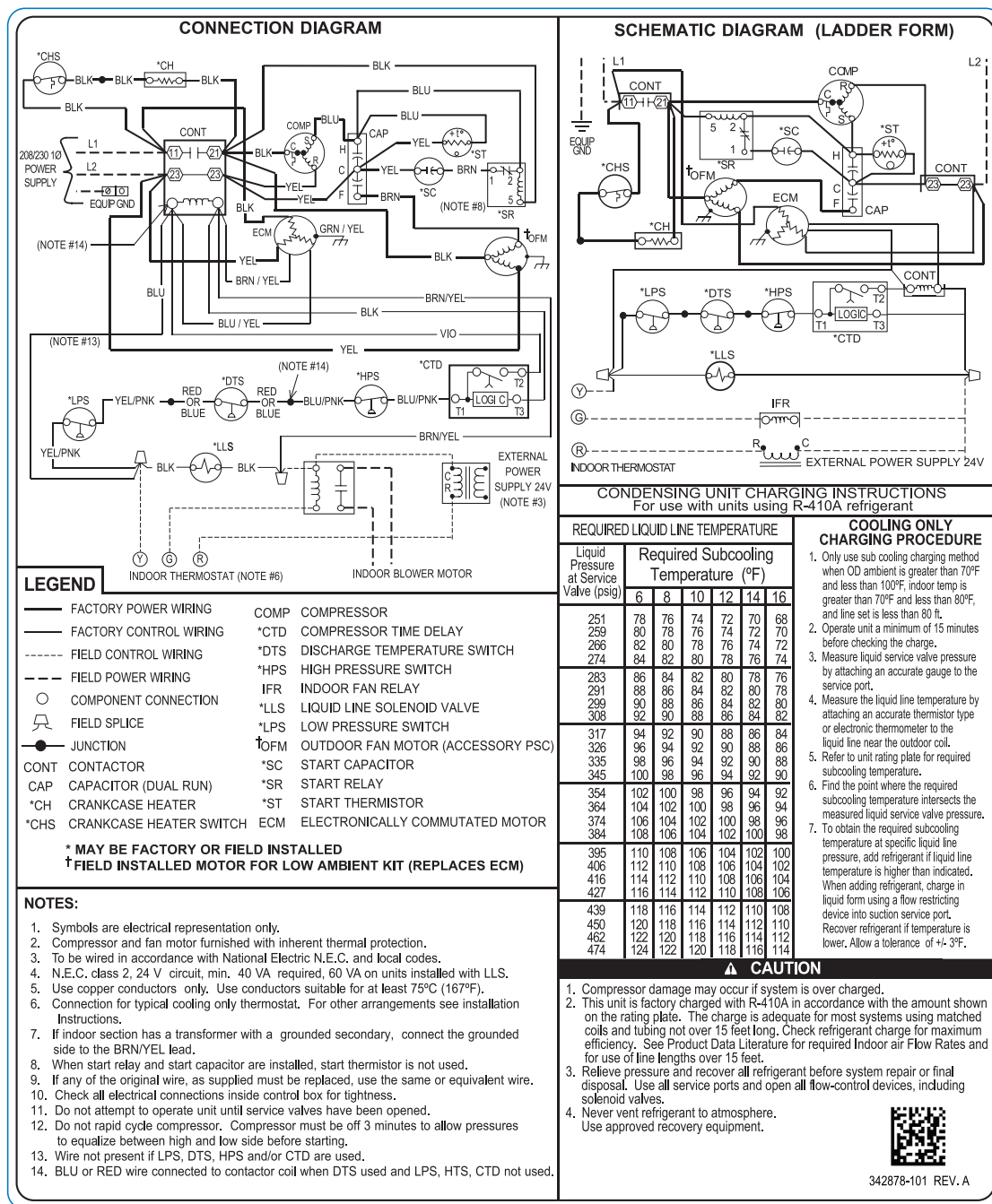
Fig. 1 – 116BNA060, 208/230-1
