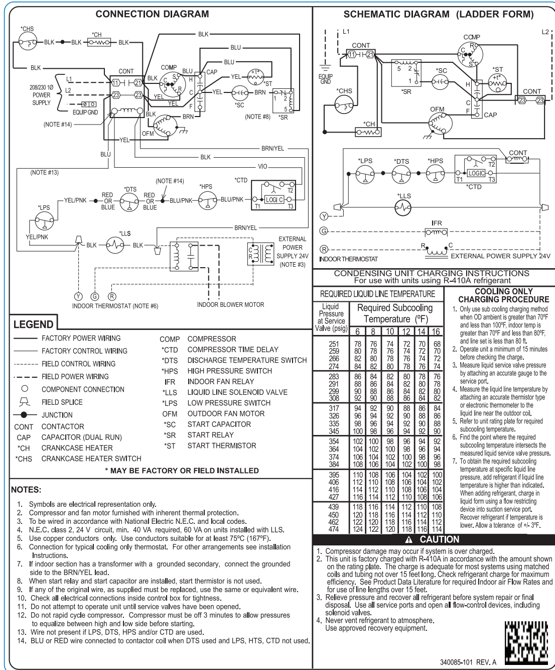
Fig. 1 – 116BNA018-48, 208/230-1
