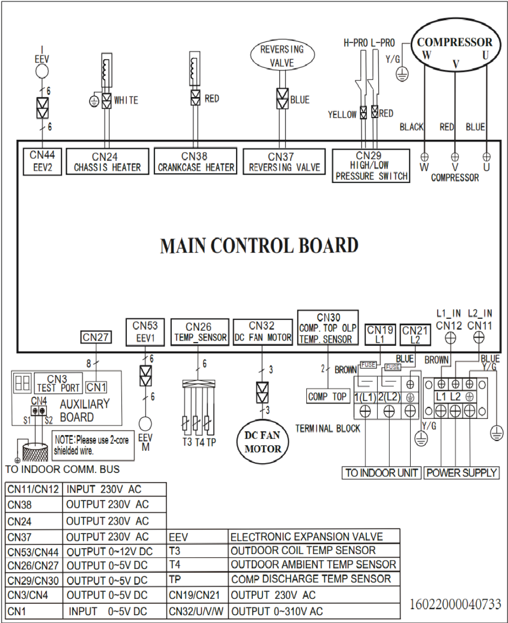
Fig. 6 – 36K Wiring Diagram
