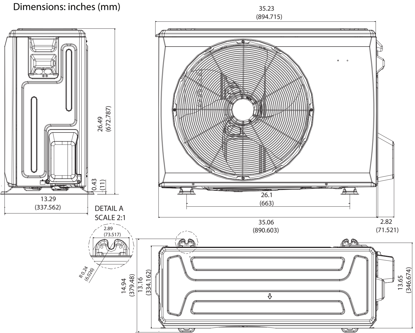
Fig. 3 — Sizes 18K / 24K
