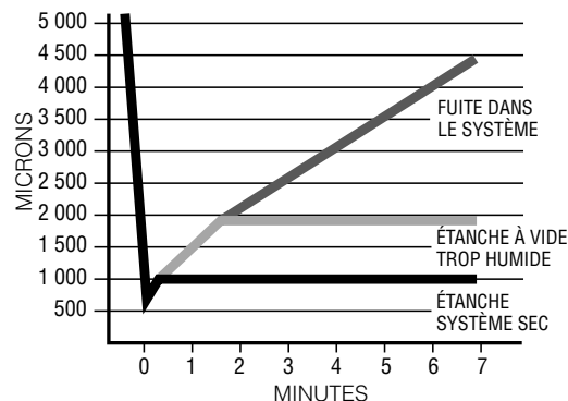
Fig. 4 – Courbe de vide A95424FR
