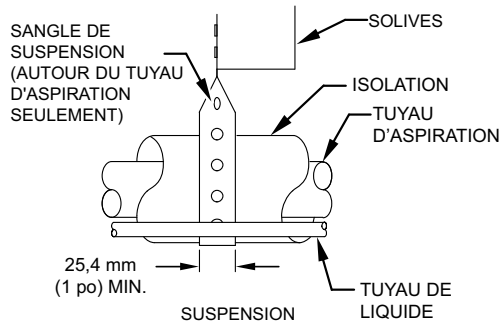
Fig. 1 – Installation de la tuyauterie
