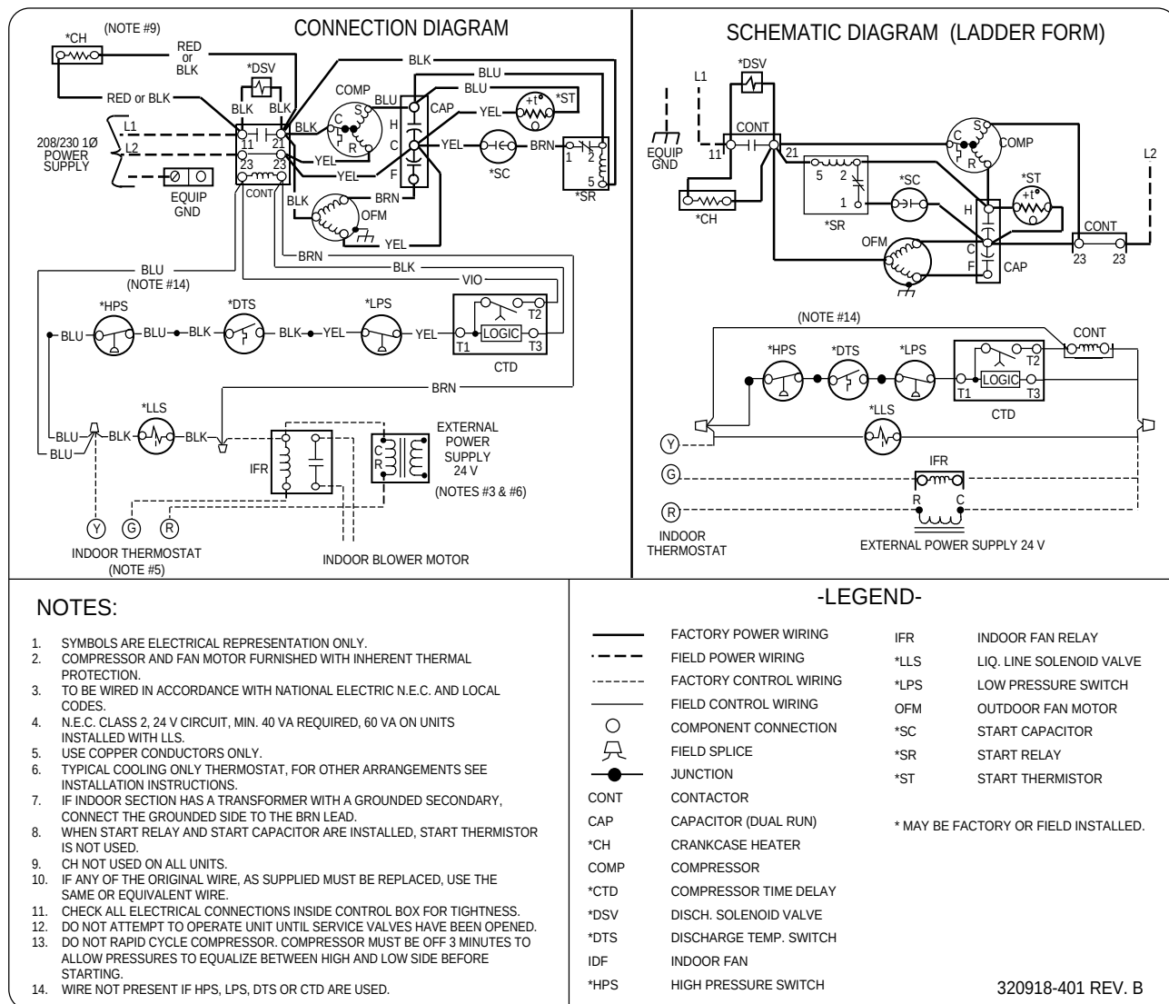
Fig. 1—594D018-048 208/230v, 1 Phase, 60 Hertz
