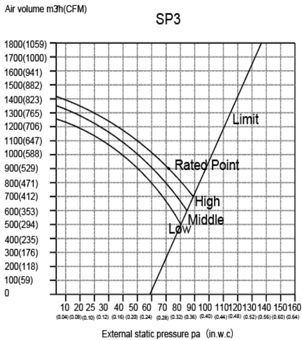
Fig. 15 — Fan Performance - DLFSDAH18XAK
