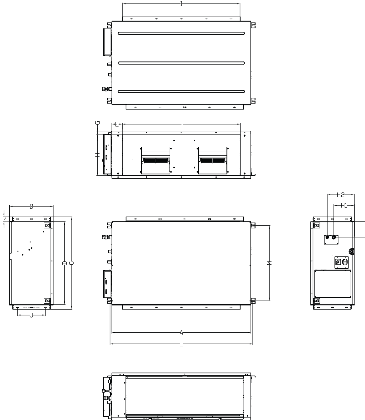
Fig. 4 — Indoor Unit Size 58K
