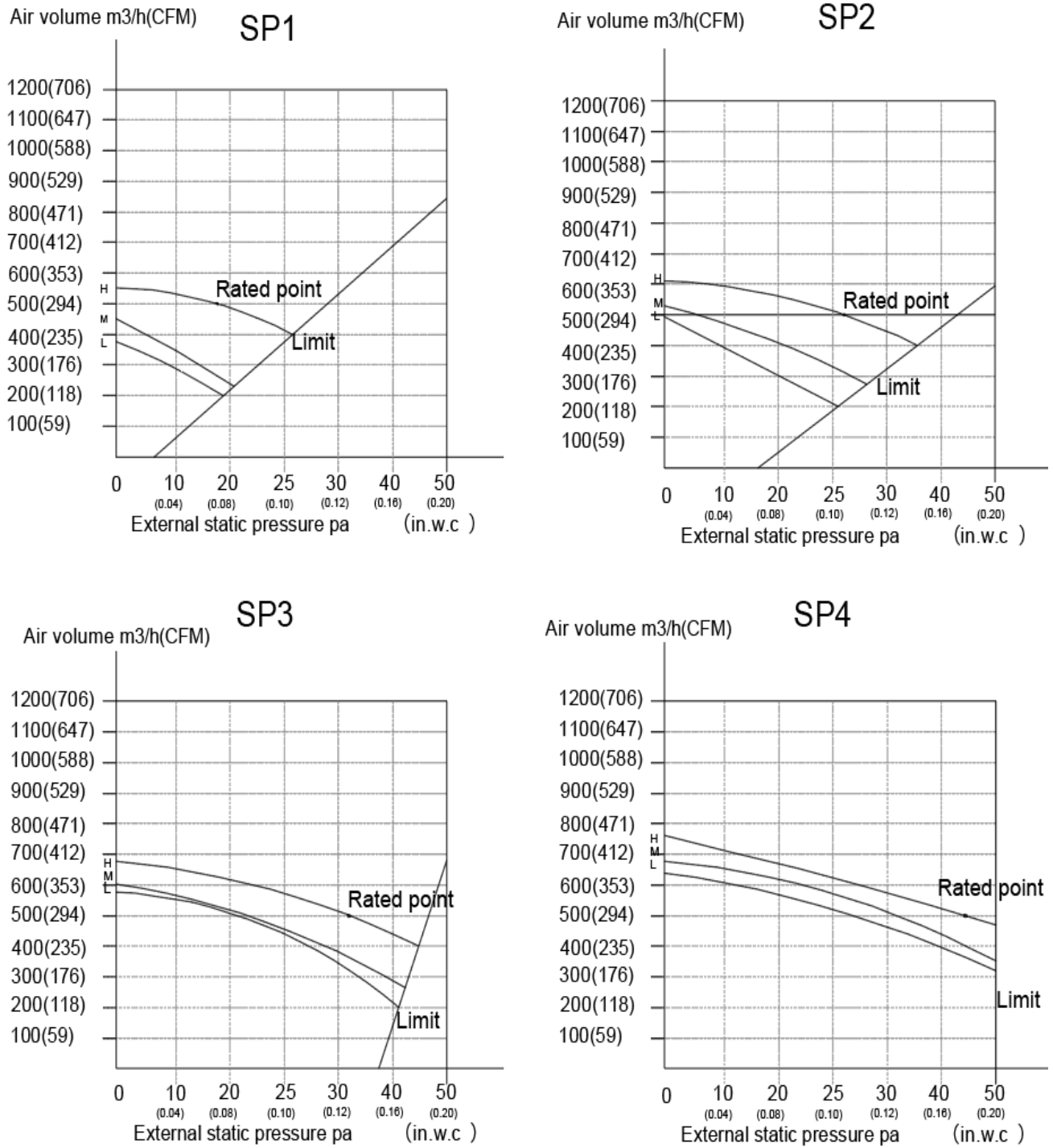
Fig. 13 — Fan Performance - DLFSDAH09XAK
