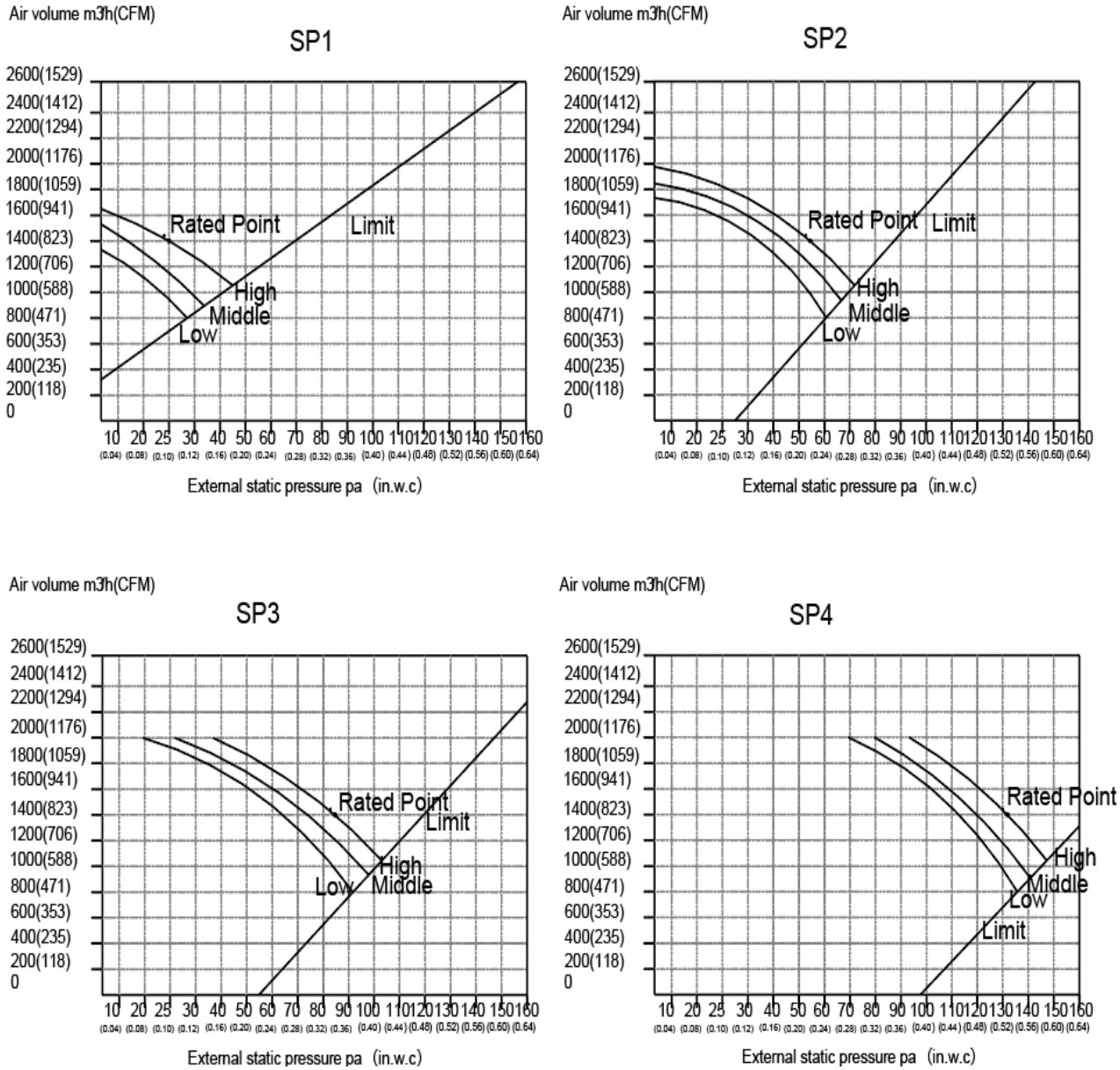
Fig. 16 — Fan Performance - DLFSDAH24XAK
