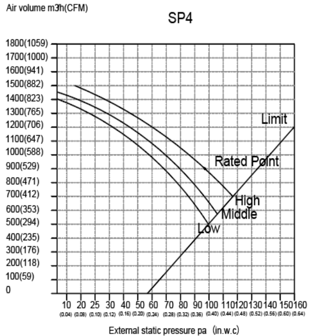
Fig. 15 — Fan Performance - DLFSDAH18XAK
