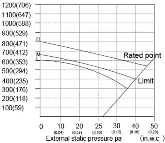
Fig. 14 — Fan Performance - DLFSDAH12XAK
