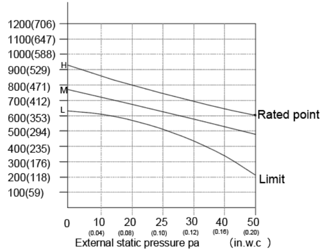
Fig. 14 — Fan Performance - DLFSDAH12XAK
