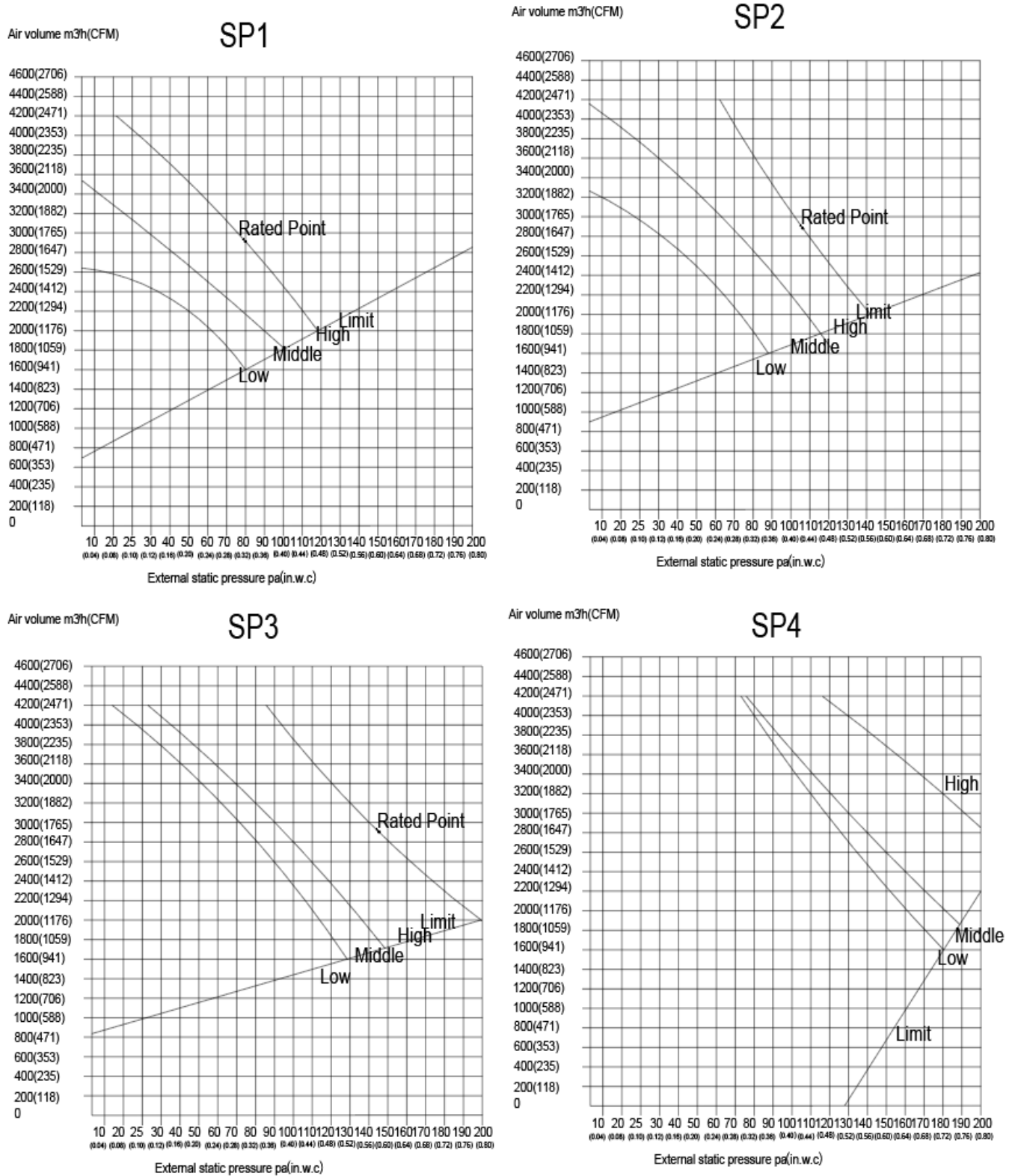
Fig. 19 — Fan Performance - DLFLDAH58XAK
