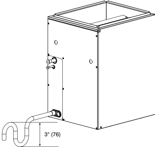
Fig. 6 - Condensate Trap
