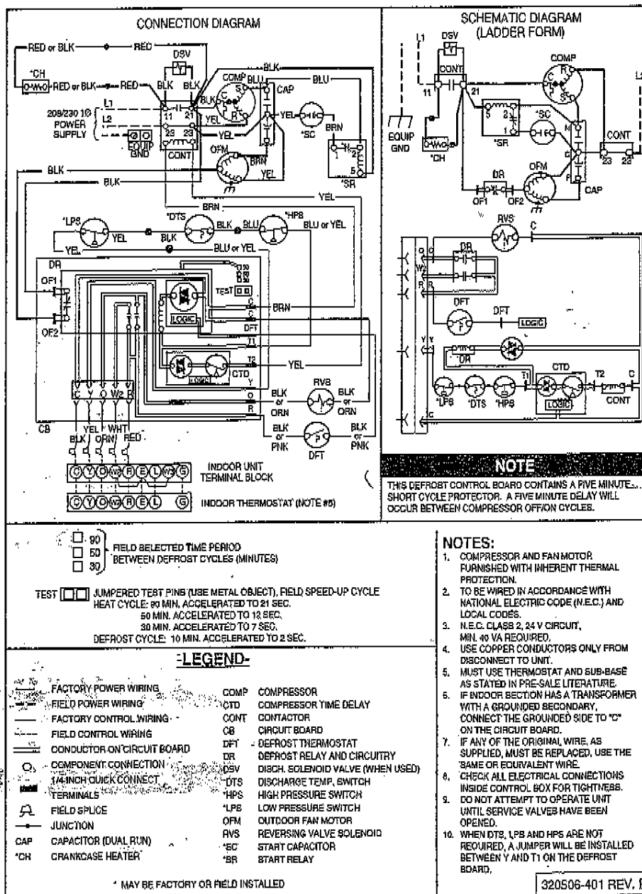
Fig. 1—PH12NA 018-A—048-A 208/230v, 1 Phase, 60 Hertz
