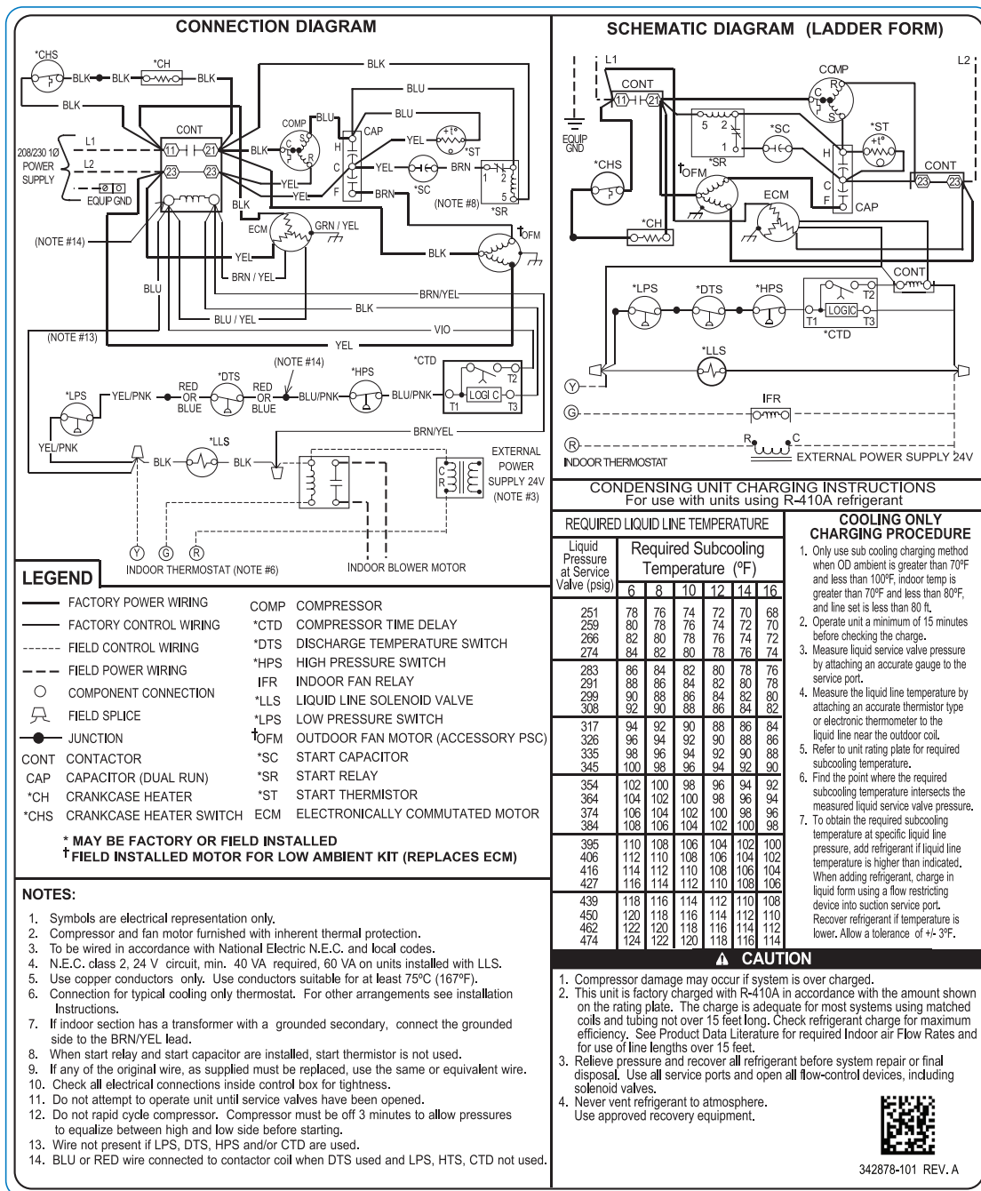
Fig. 1 – 105ANA061, 208/230-1
