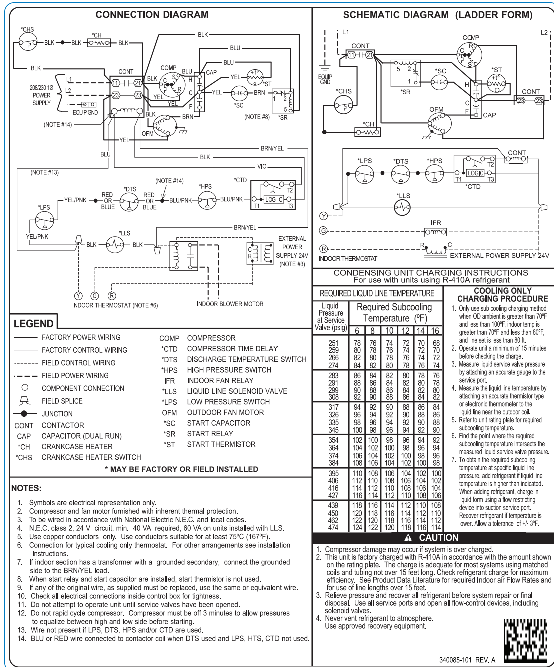
Fig. 1 – 105ANA018-60 / 106ANA018-60, 208/230-1
