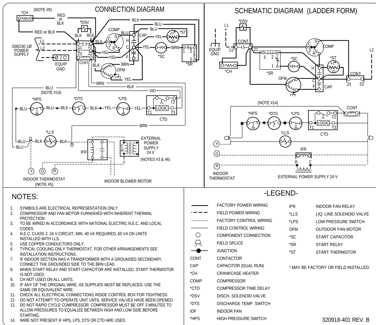
Fig. 1—38TUA018-048 (0,1) 208/230v, 1 Phase, 60 Hertz
