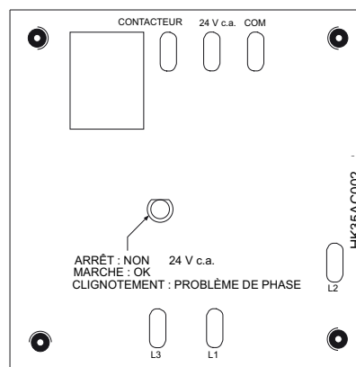
Figure 6 – Commande de moniteur triphasé (s'applique aux appareils triphasés seulement)
