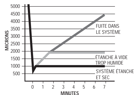
Figure 4 – Schéma du vide poussé
