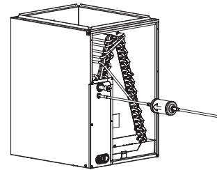
Figure 3 – Déshydrateur-filtre de la conduite de liquide Évacuer les tuyaux de frigorigène et le serpentin intérieur
