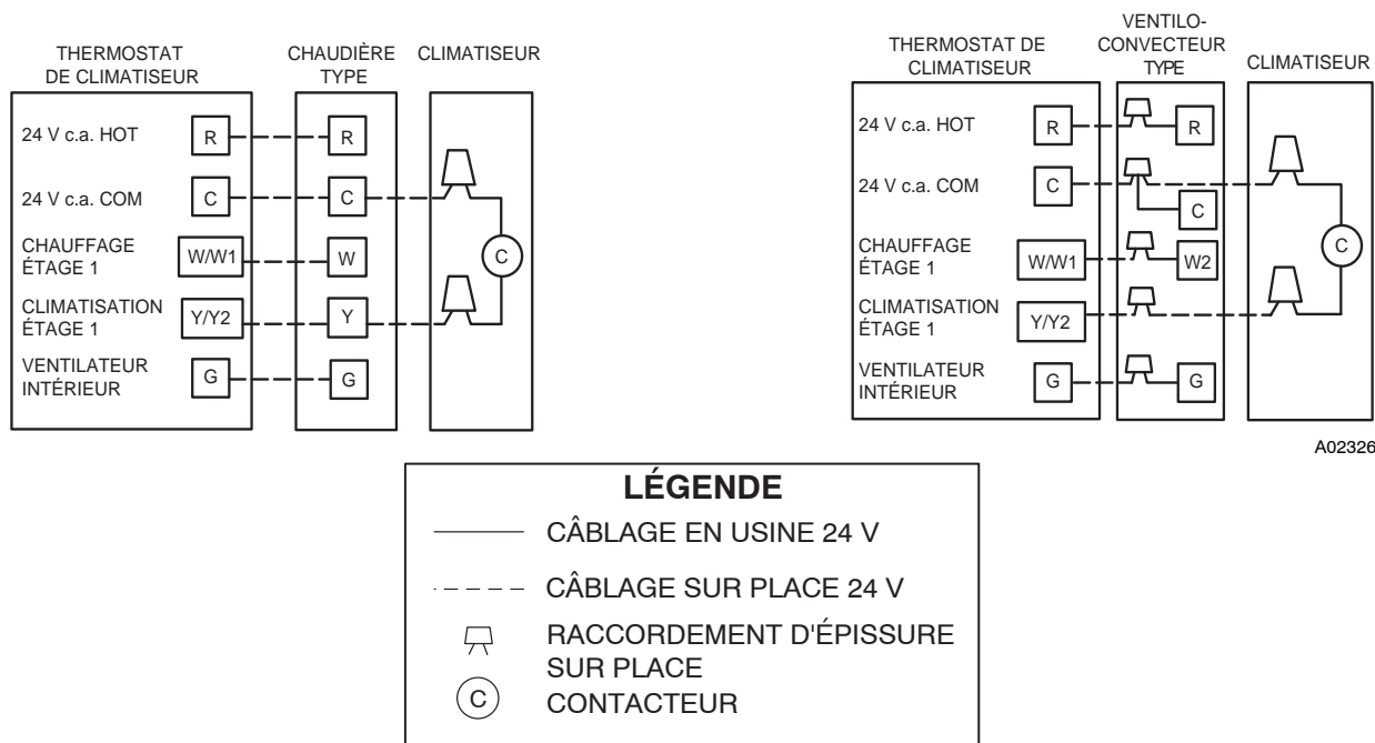
Figure 7 – Schémas de câblage génériques (consultez les instructions d'installation du thermostat pour connaître les combinaisons spécifiques des appareils)
