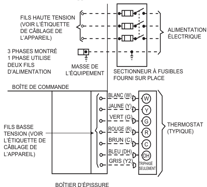
Fig. 10 – Branchements haute et basse tensions
