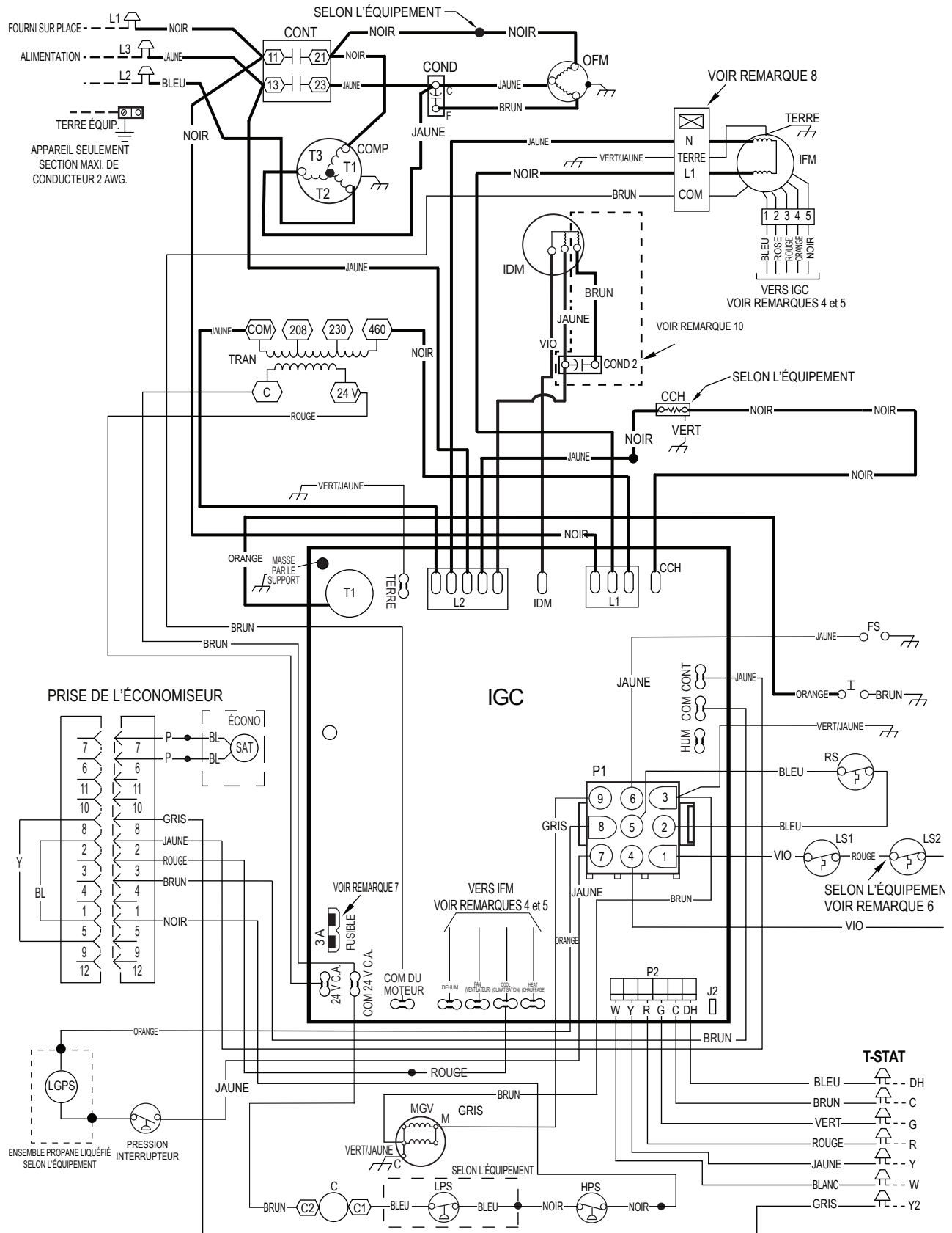
Fig. 18 – Schéma de connexion de câblage – 460-3-60
