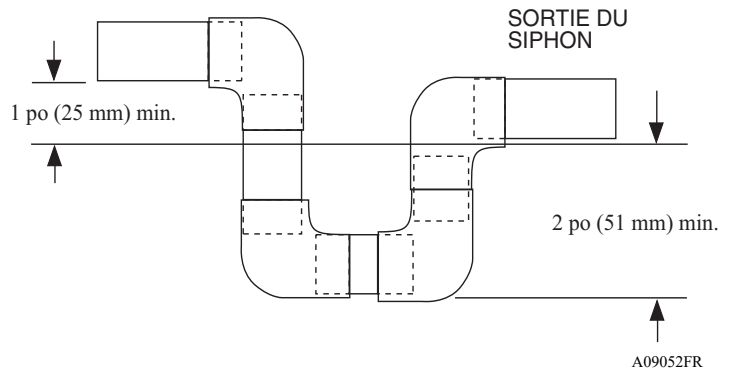
Fig. 7 – Siphon de condensat
