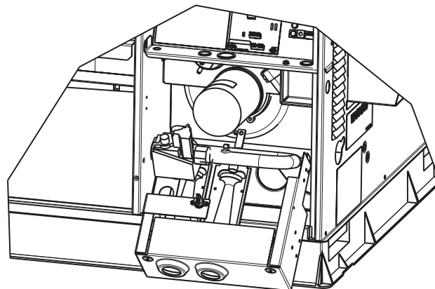
Fig. 24 – Porte-brûleur déposé
