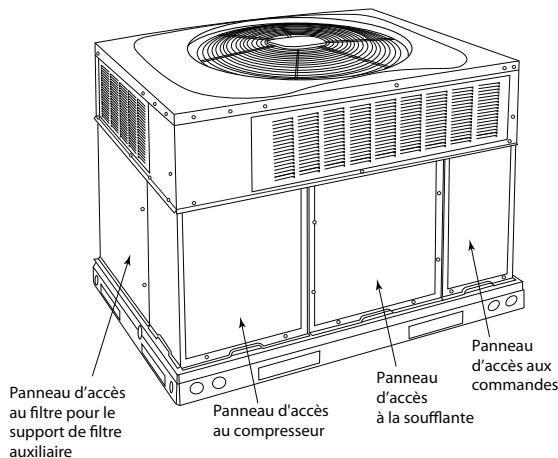
Fig. 22 – Panneaux d'accès de l'appareil
