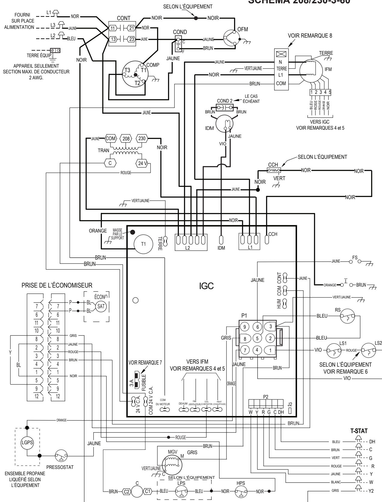
Fig. 16 – Schéma de connexion de câblage – 208/230-3-60
