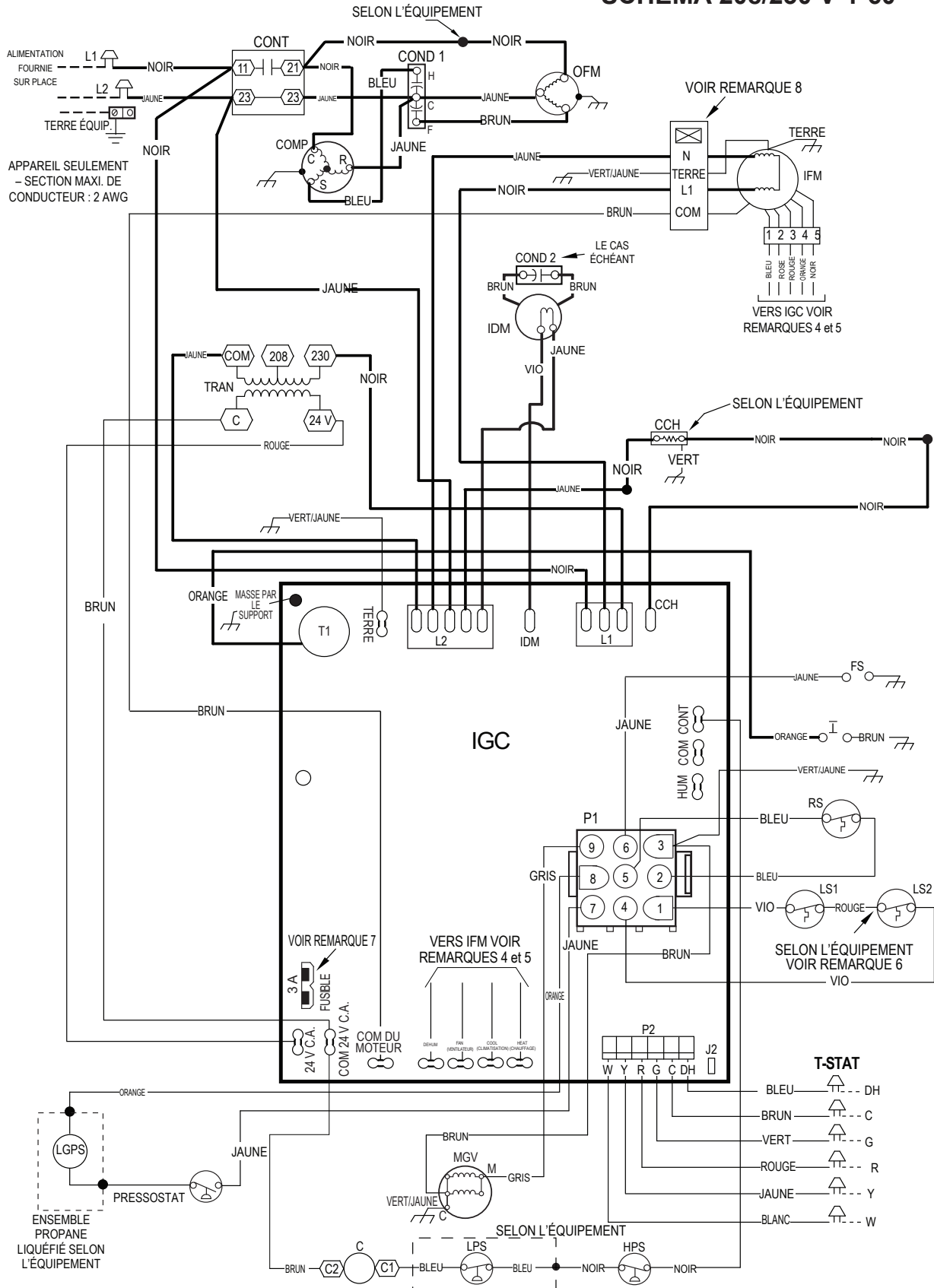
Fig. 14 – Schéma de connexion de câblage – 208/230 V, 1 phase, 60 Hz
