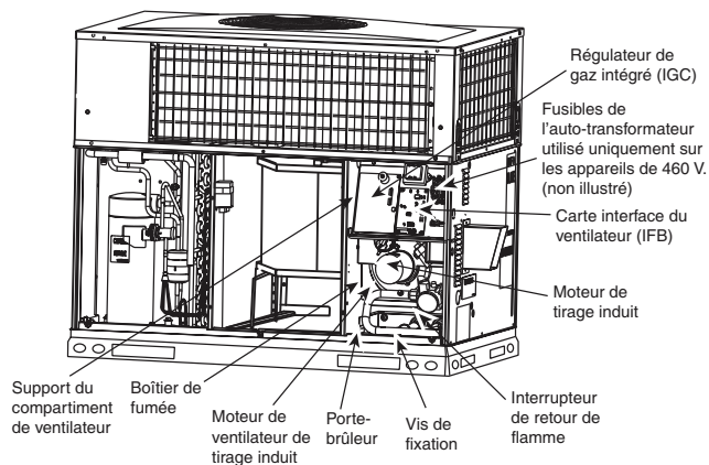
Fig. 21 – Compartiment de ventilateur et boîtier de fumée
