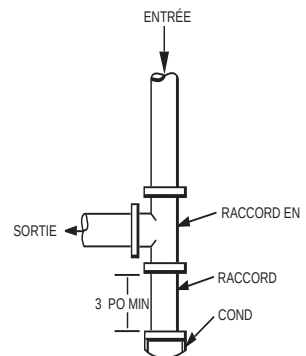
Fig. 8 – Piège à sédiments
