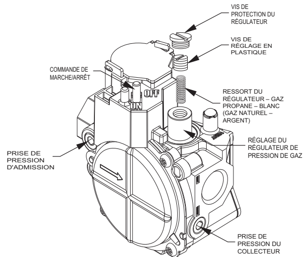
Fig. 13 – Vanne de gaz à une phase
