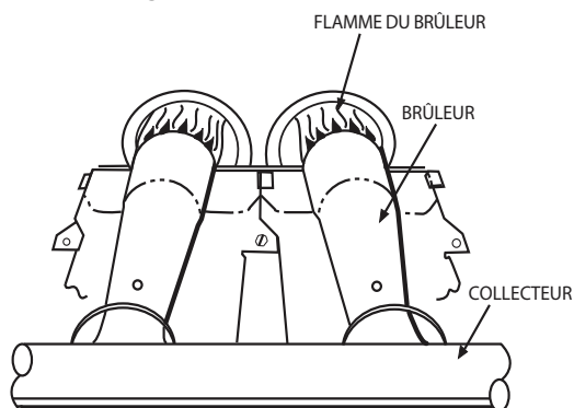
Fig. 12 – Brûleur monoport
