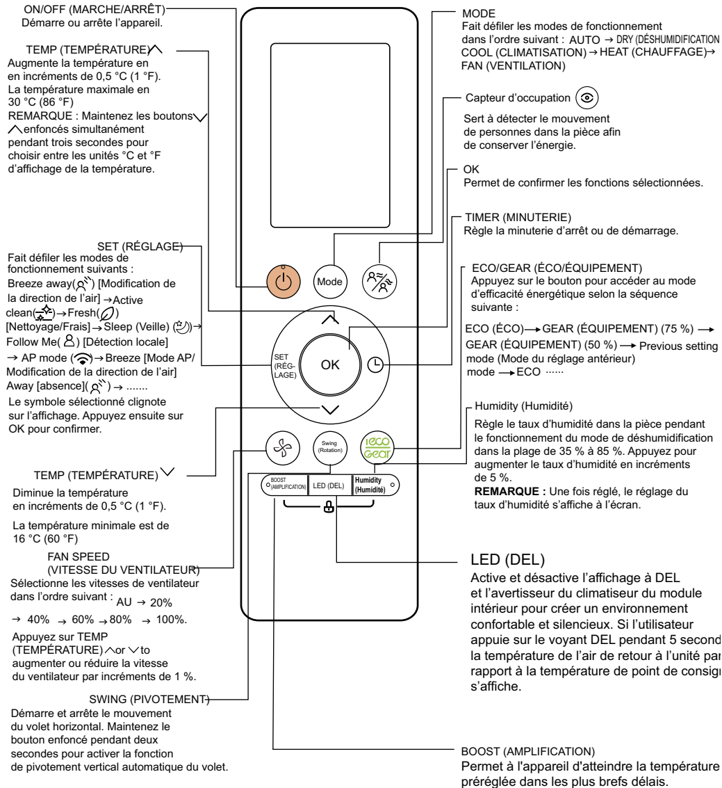
Fig.2 –Fonctions de la télécommande
