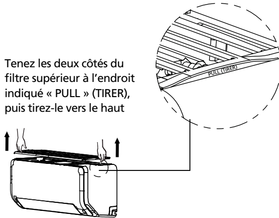
Fig.18 –Maintenir et tirer le filtre
