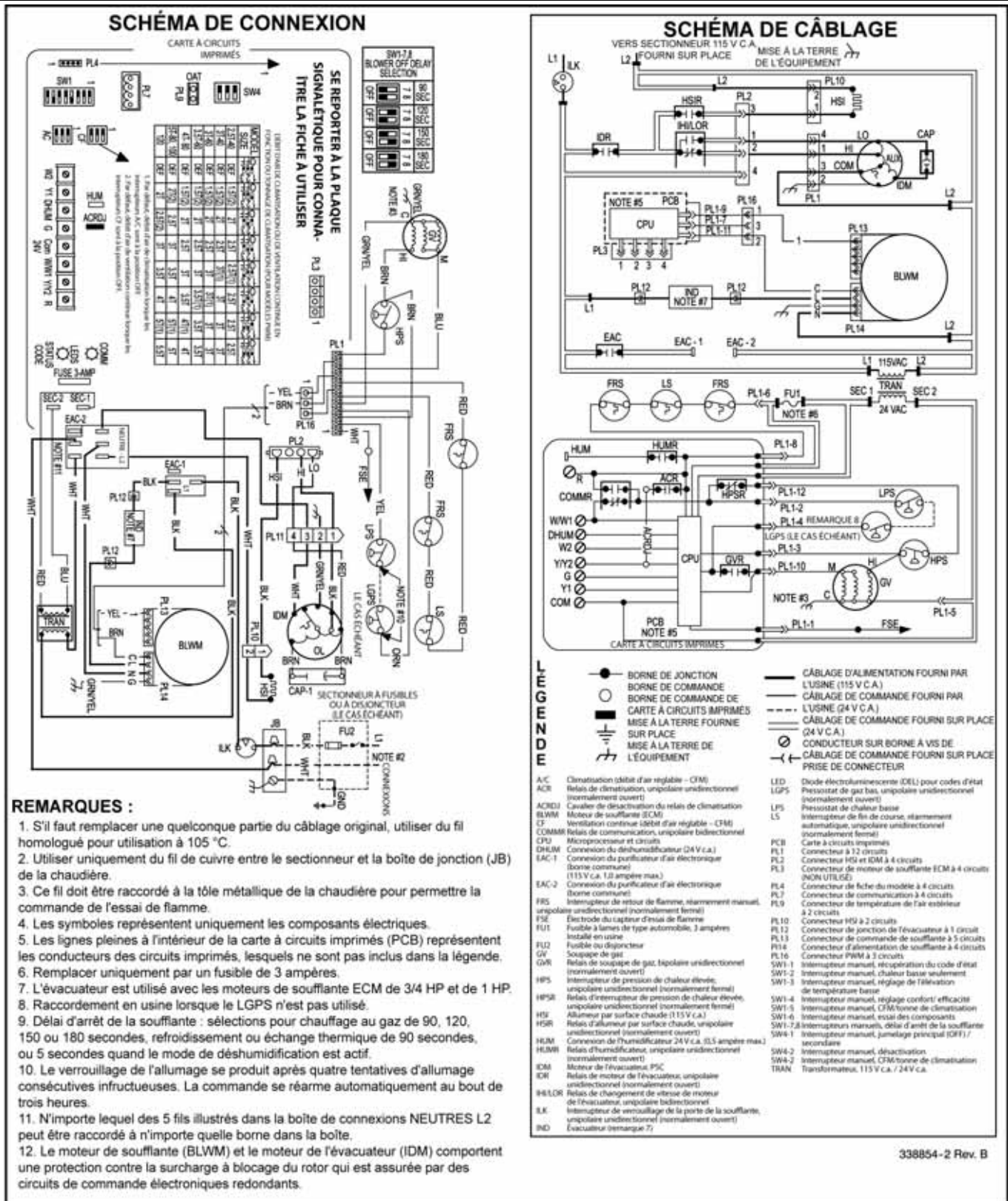
Figure 16 Schéma de câblage
