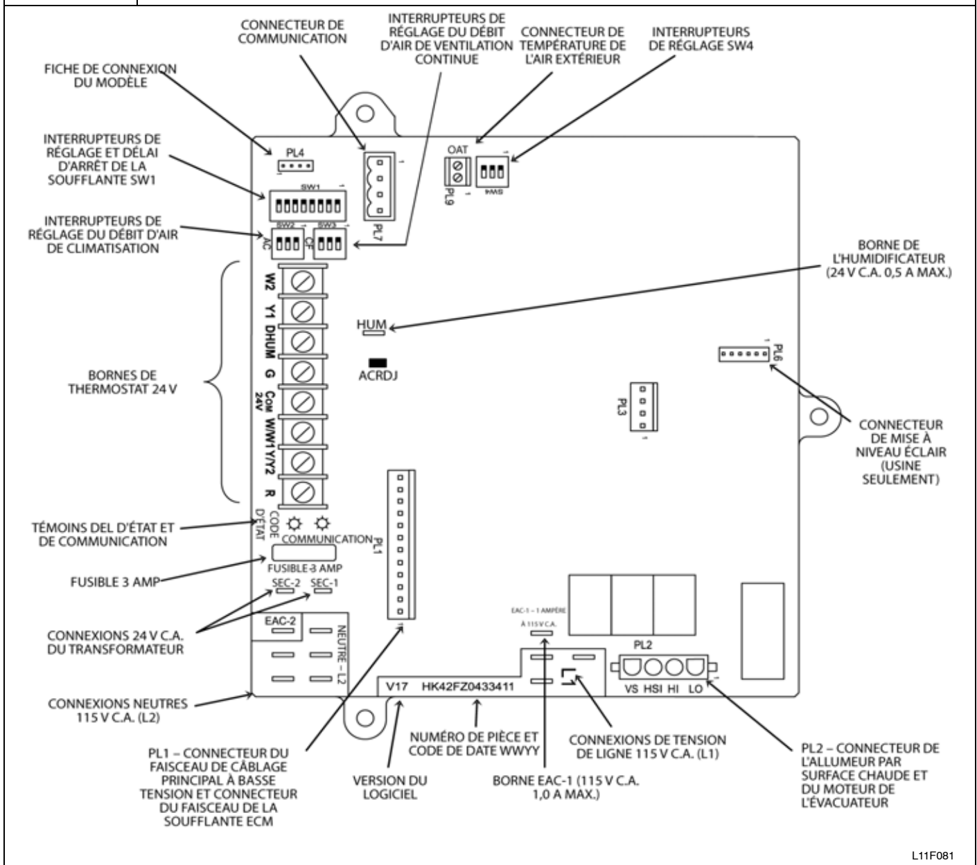
Figure 4 Exemple de commande de chaudière à vitesse variable pour moteur de soufflante ECM
