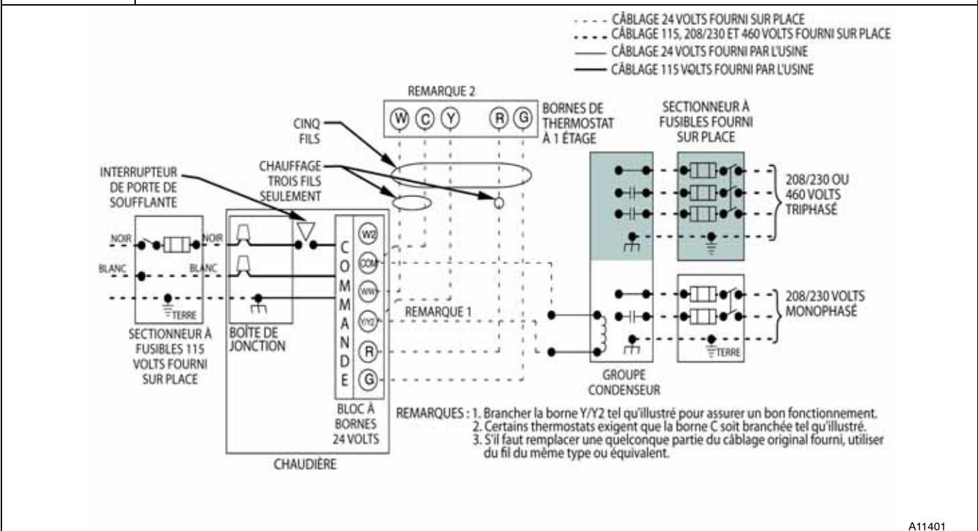
Figure 8 Schémade câblage du chauffage et de la climatisation – Thermostat à étage unique
