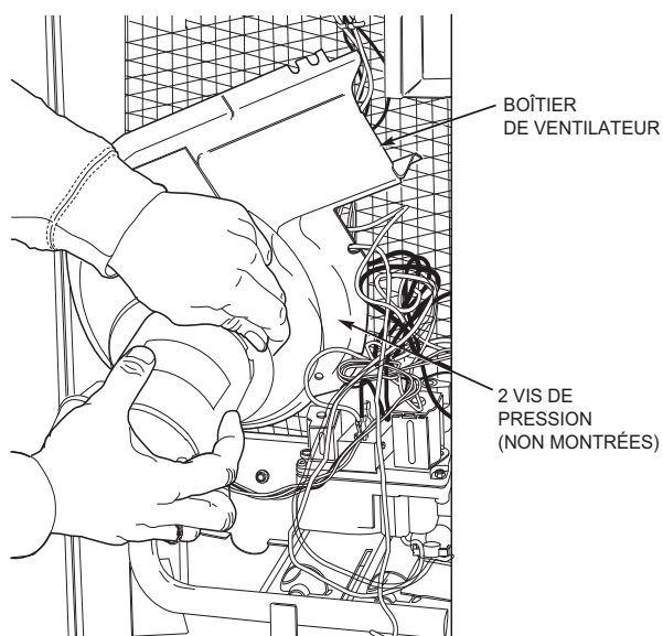
Figure 22 – Retrait du moteur et de la roue de ventilateur
