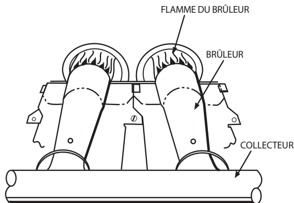
Figure 14 – Brûleur monoport
