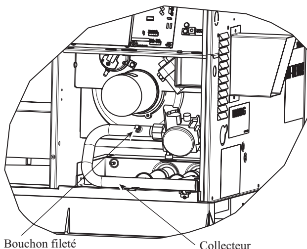
Figure 13 – Ensemble de brûleur
