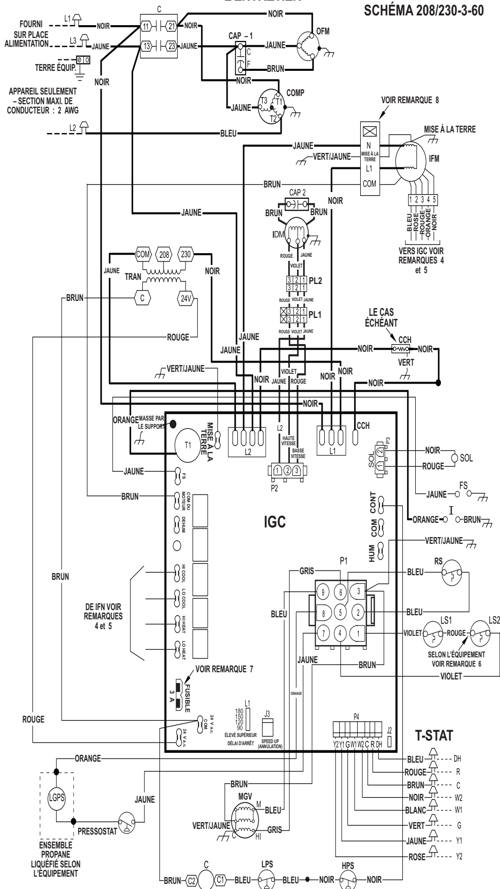
Figure 17 – Modèles 208/230 V 3 phases 60 Hz Schéma de connexion de câblage, pouvoirs calorifiques 40, 60 et 90 KBtu/h
