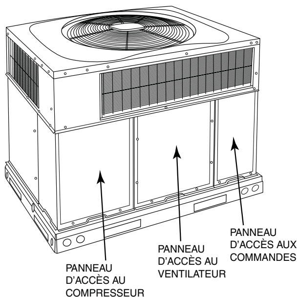
Figure 21 – Panneaux d'accès de l'appareil
