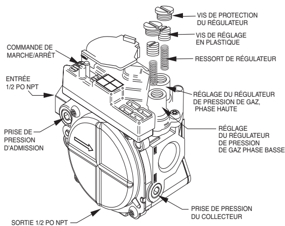
Figure 15 – Vanne de gaz à deux étages
