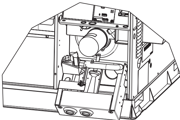
Figure 23 – Porte-brûleur déposé
