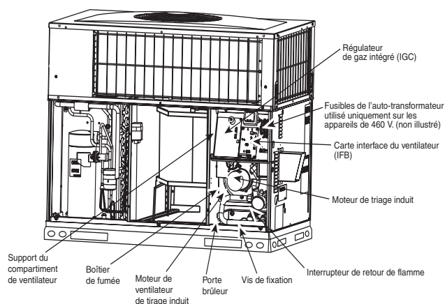
Figure 20 – Compartiment de ventilateur et boîtier de fumée
