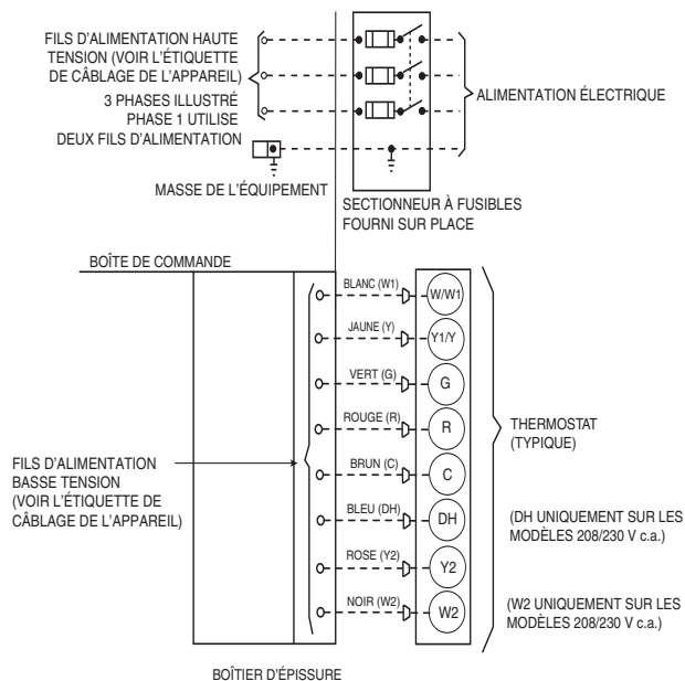
Figure 12 – Branchements haute et basse tensions
