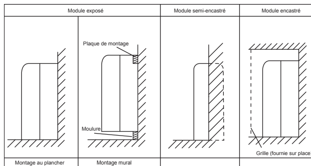
Figure 41 – Schémas d'installation du module intérieur
