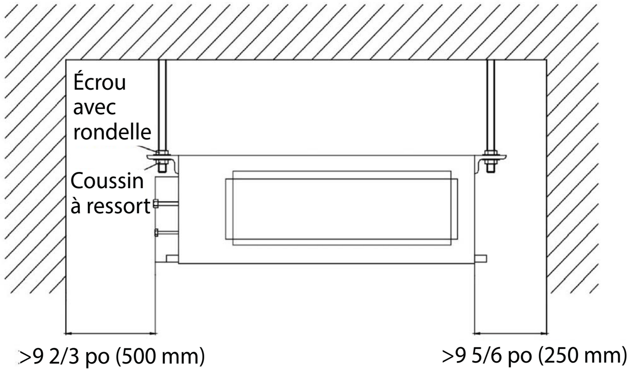
Figure 16 – Déagements – système de conduites
