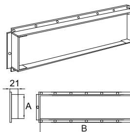
Figure 32 – Sortie d'alimentation d'air
