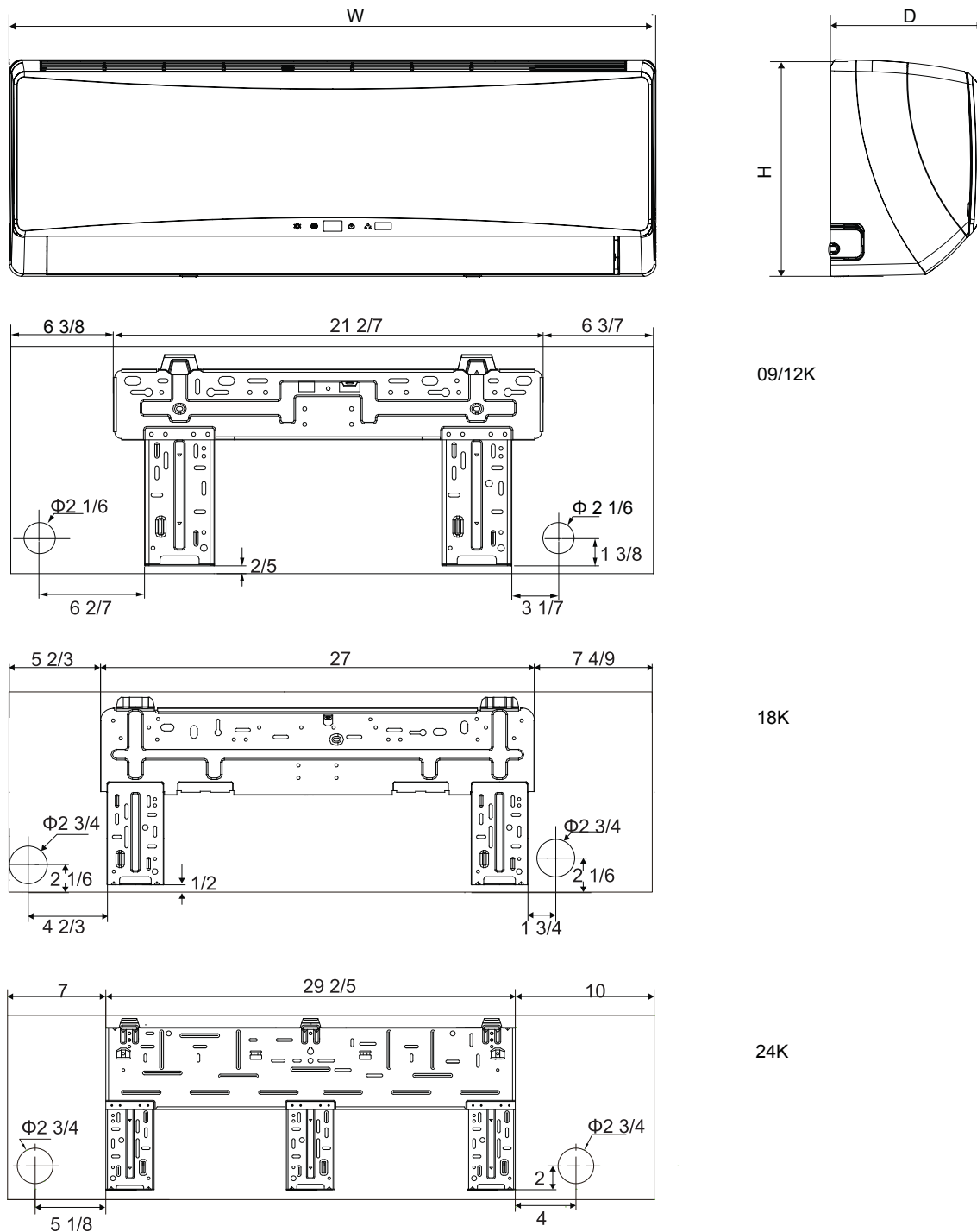
Figure 3 – Dimensions du mur
