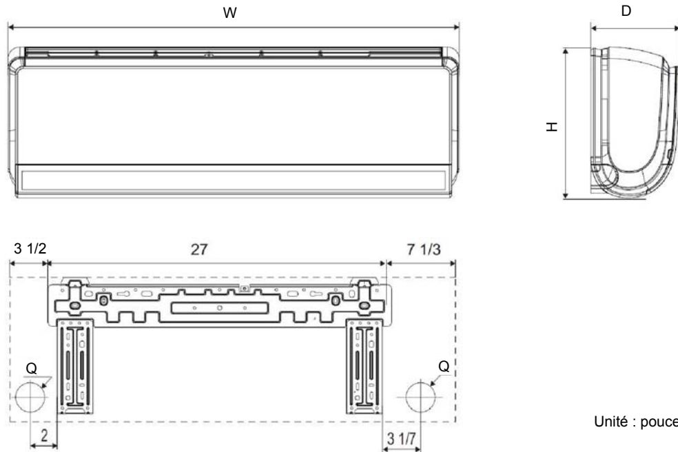
Figure 2 – Dimensions du montage en hauteur
