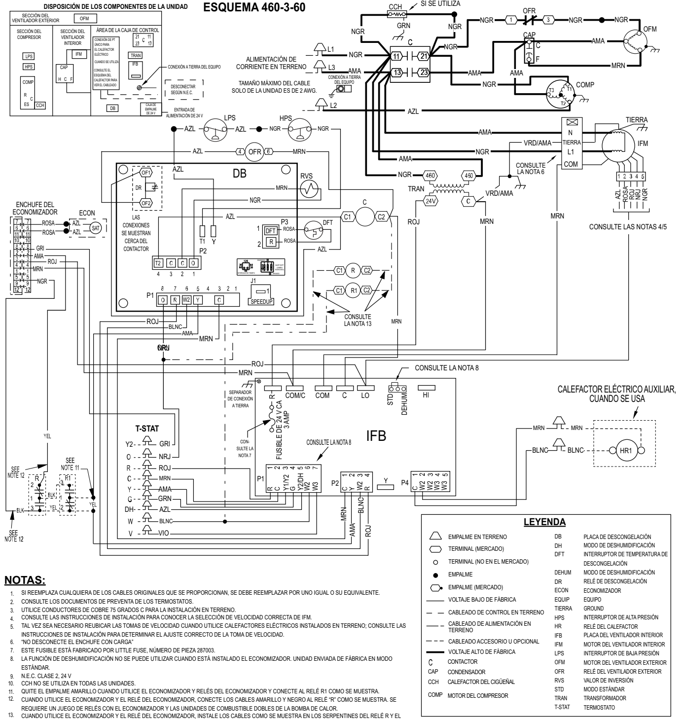
Fig. 18 – Diagrama eléctrico de conexión 460-3-60
