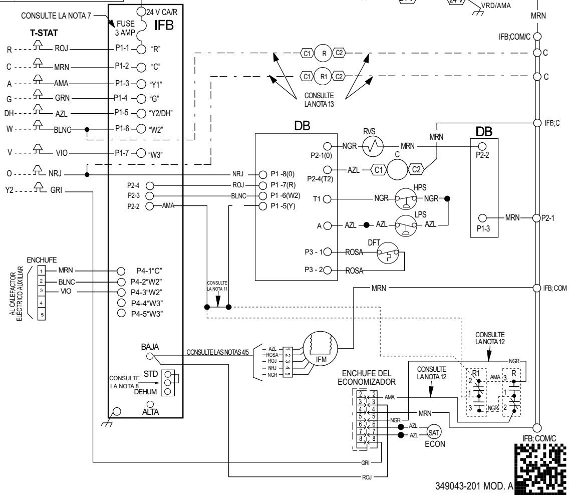
Fig. 17 – Esquemas del cableado escalera - 208/230-3-60
