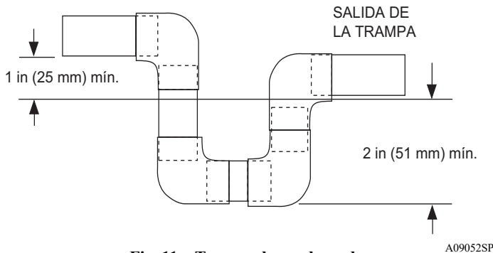
Fig. 11 – Trampa de condensado
