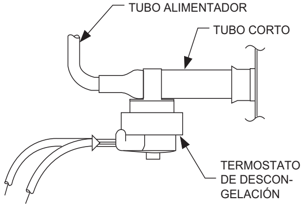
Fig. 27 – Termostato de descongelación
