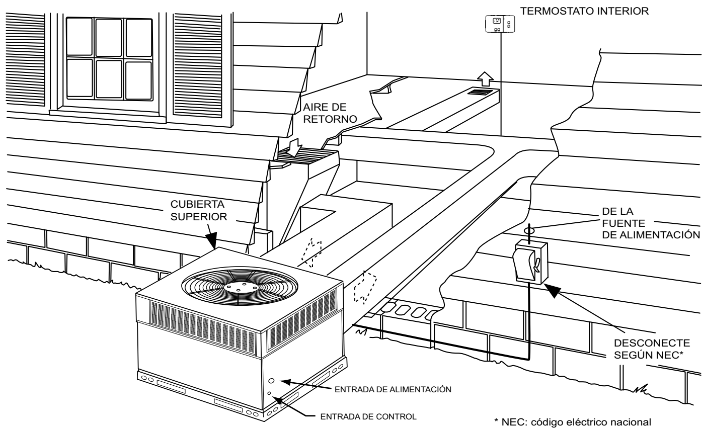
Fig. 13 – Instalación típica
