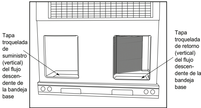
Fig. 8 – Abertura del conducto de alimentación y retorno
