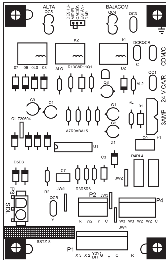
Fig. 21 – Placa de la interfaz del ventilador (IFB)
