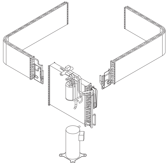
Fig. 24 – Circuito de refrigerante
