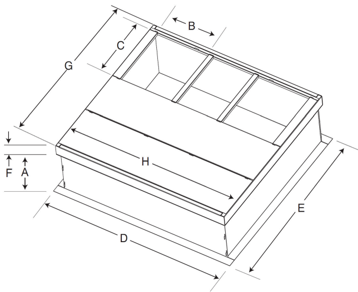
Fig. 6 – Dimensiones del bordillo del techo
