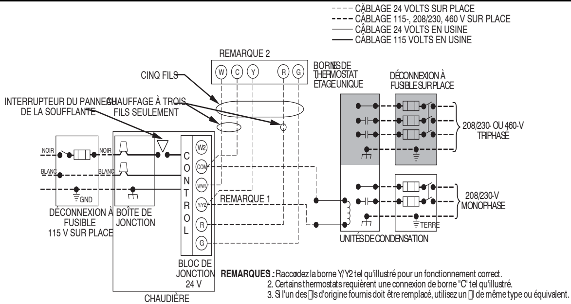
Figure 8 Schéma de câblage de site à deux étages type
