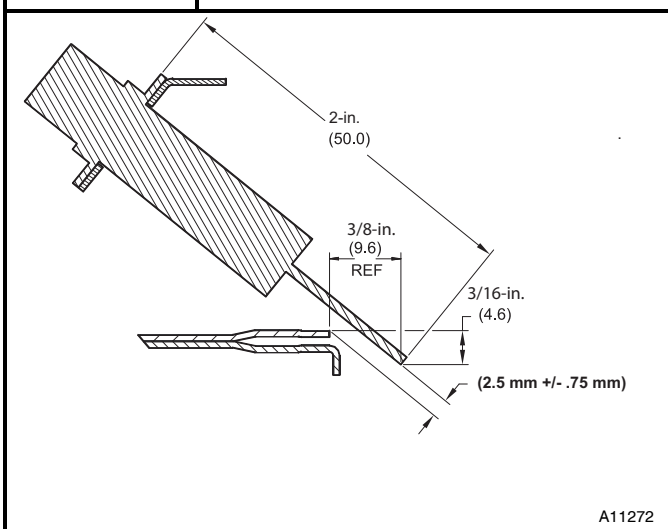
Figure 12 Position de l'allumeur - vue latérale
