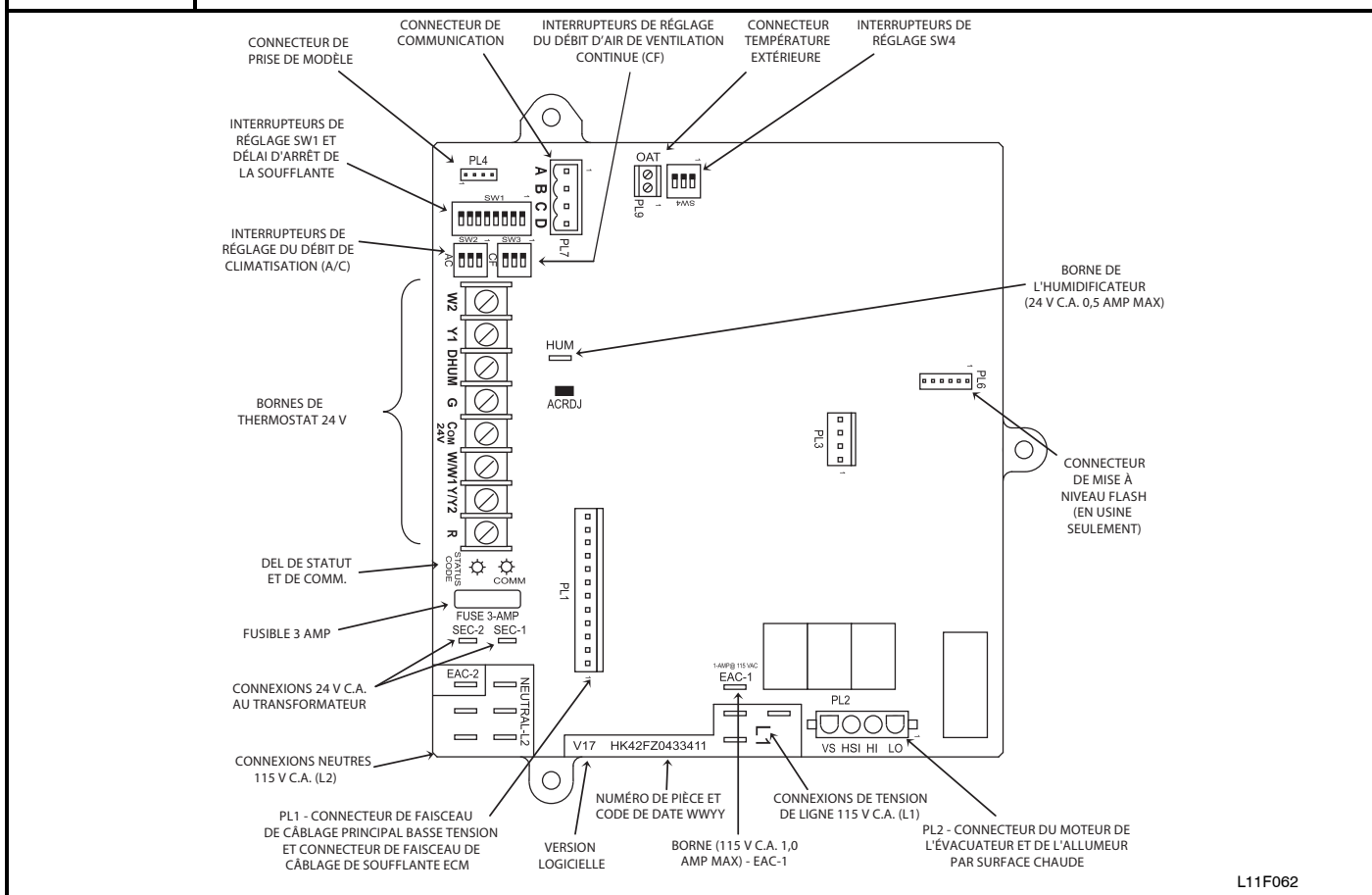
Figure 4 Commande de chaudière à vitesse variable pour moteur de soufflante ECM
