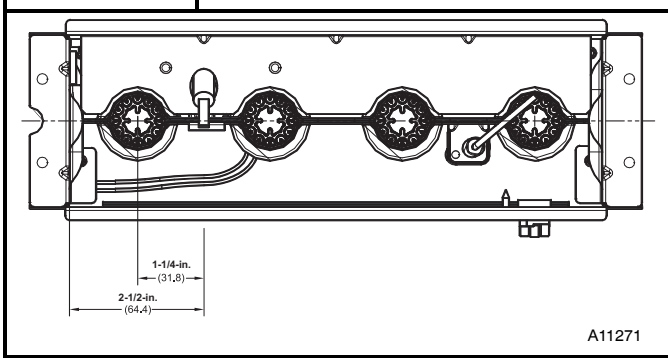
Figure 11 Position de l'allumeur - vue du haut
