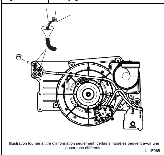
Figure 1 Amorçage du drain de condensat
