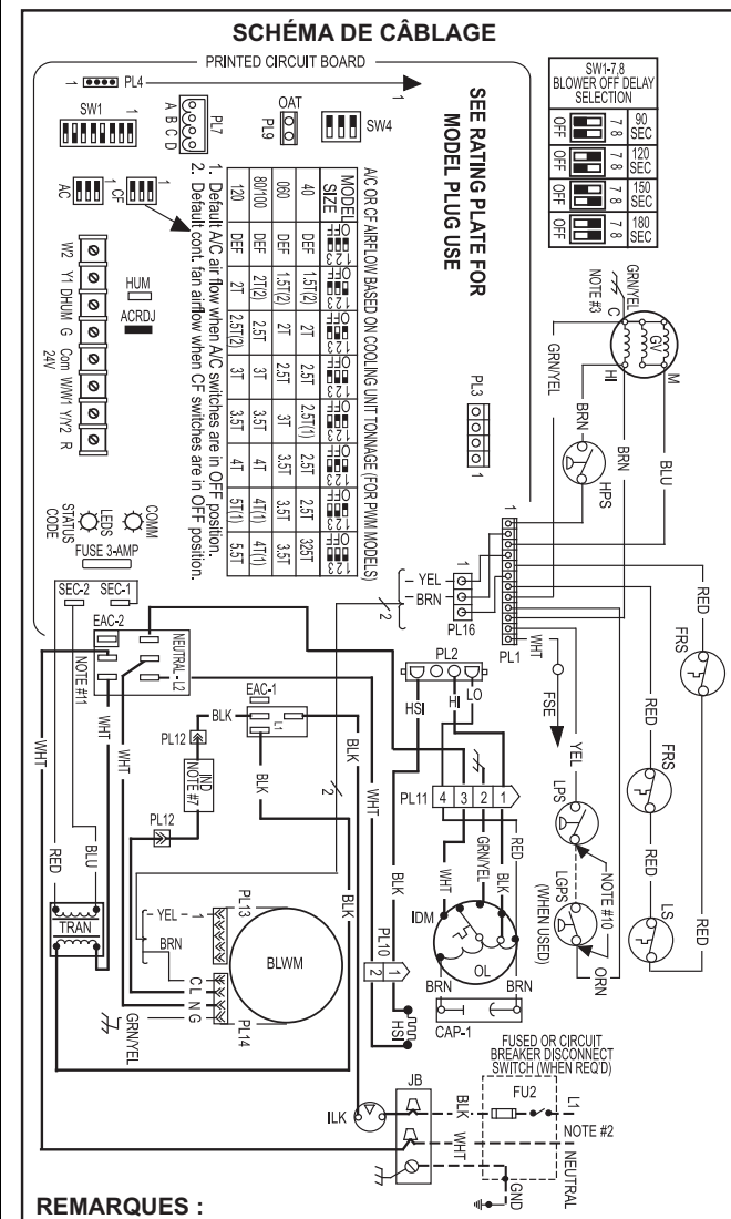
Figure 16 Schéma de câblage
