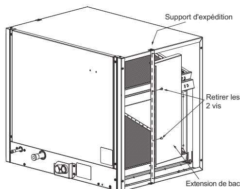
Figure 1 - Serpentin ENH4X pour appareils de chauffage
