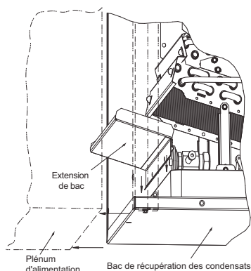
Figure 2 - Installation horizontale vers la gauche de l'extension du bac (capacités 43, 60 et 61 seulement)
