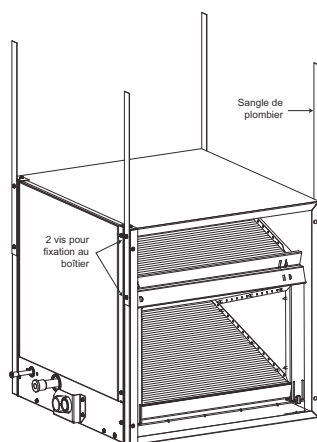
Figure 7 - Suspension du serpentin ENH4X à l'aide de feuillard perforé
