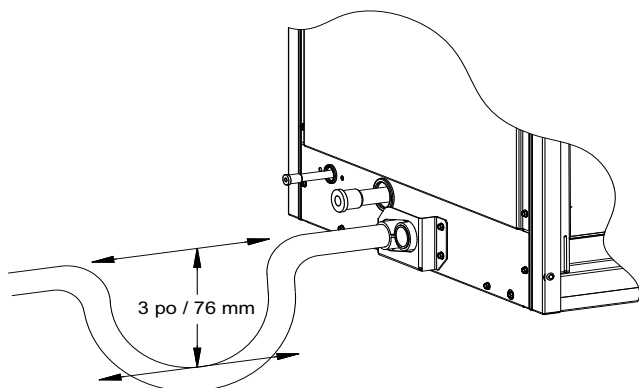
Figure 8 - Siphon de condensat
