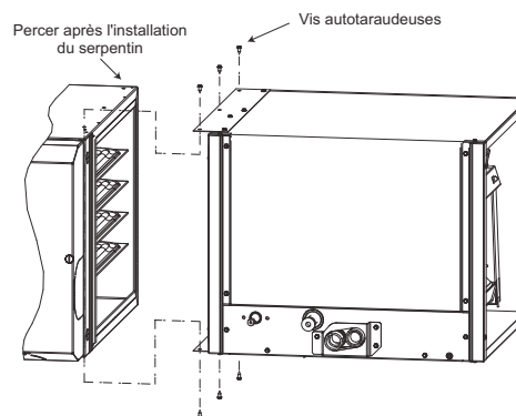
Figure 6 - Fixer le serpentín à l'appareil de chauffage
