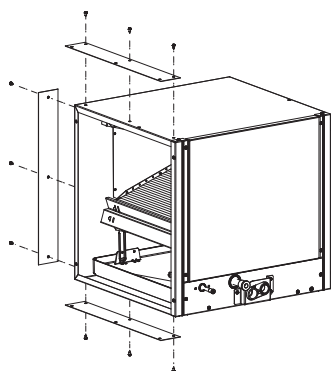
Figure 5 - Monter les plaques de fixation
