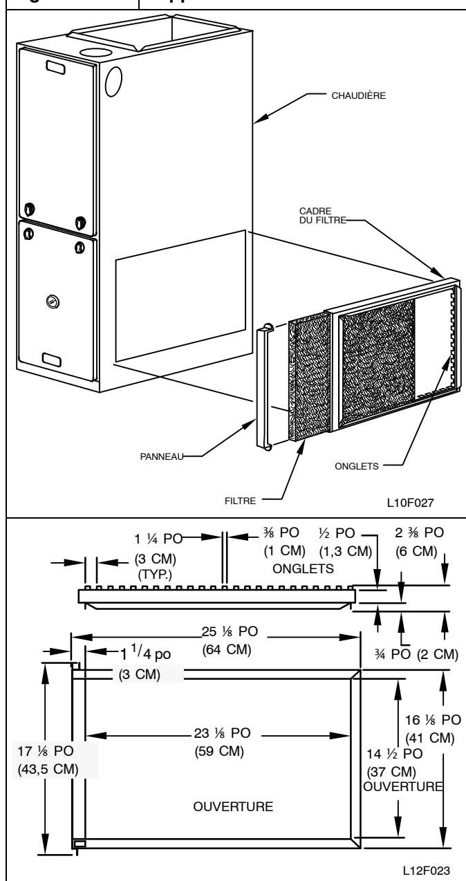
Figure 32 Support de filtre latéral
