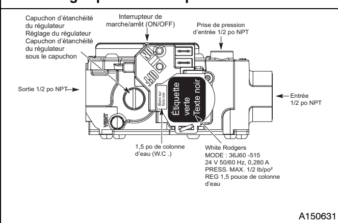
Vanne de gaz pour faible capacité de 26 000 BTUH
