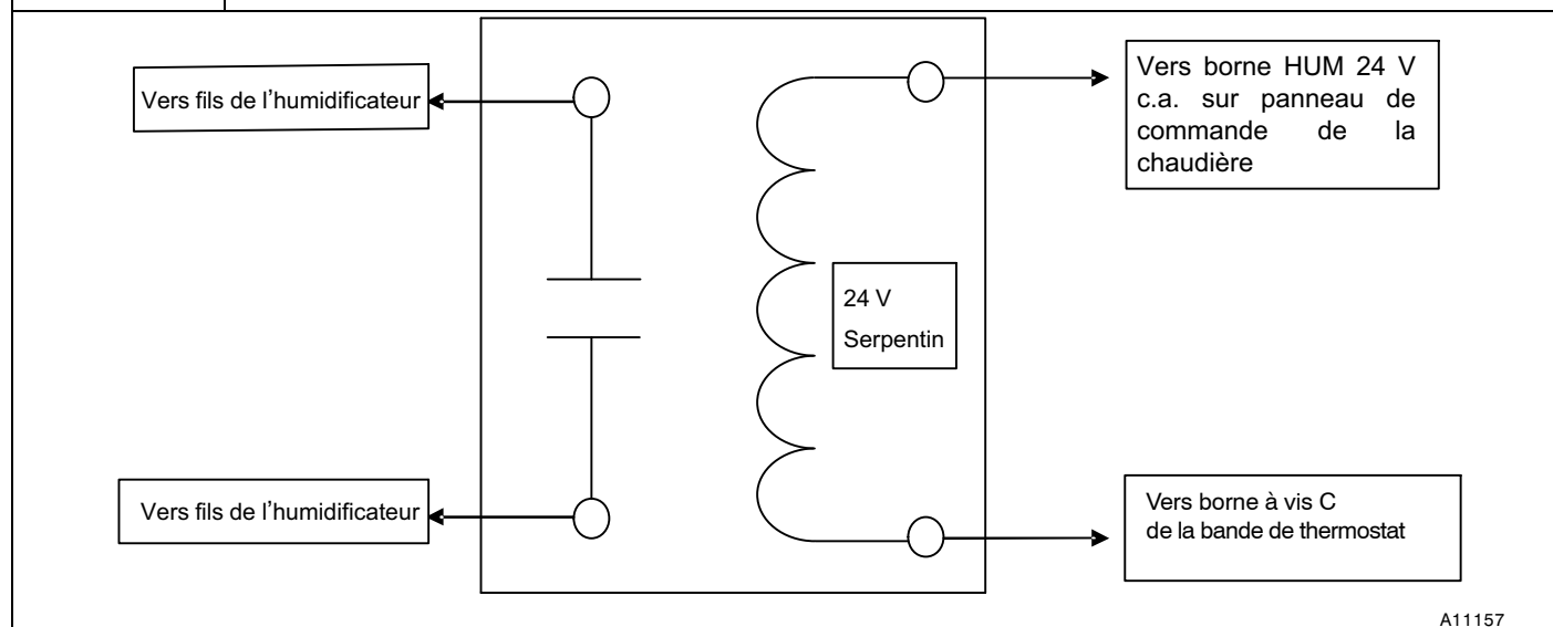
Figure 40 Relais d'isolation pour les humidificateurs dotés d'une alimentation électrique interne
