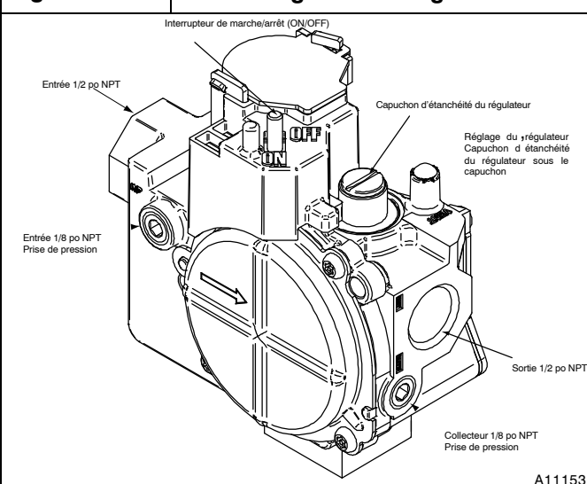
Vanne de gaz pour faible capacité de 26 000 BTUH
