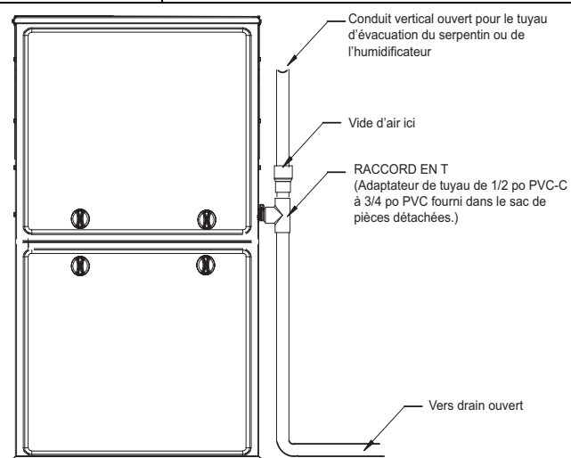
Figure 14 Exemple de fixation au tuyau d'évacuation sur place
