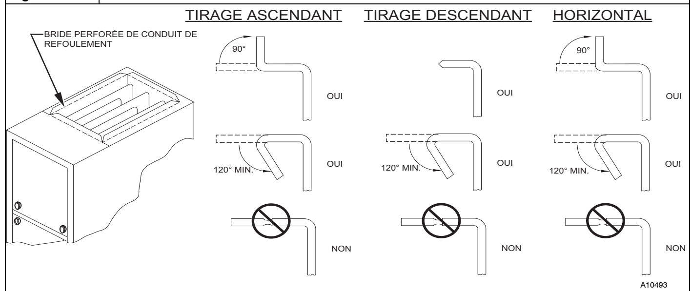
Figure 23 Brides du conduit
