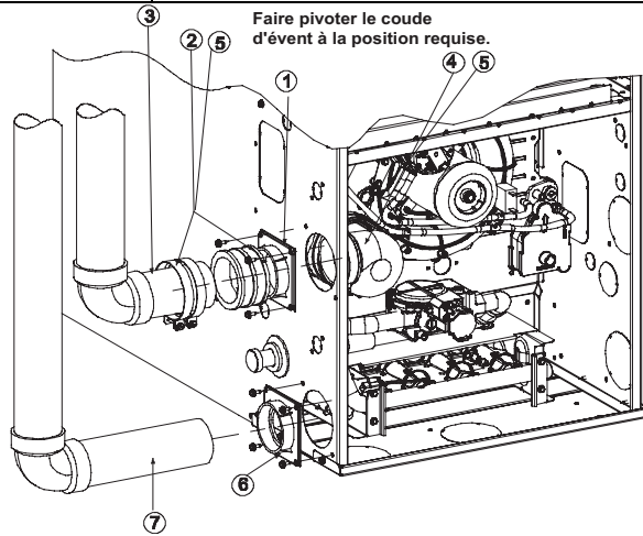
CONFIGURATION À GAUCHE À TIRAGE DESCENDANT
