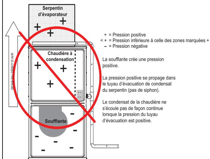
Figure 13 Exemple de fixation au tuyau d'évacuation sur place (NON AUTORISÉ)
