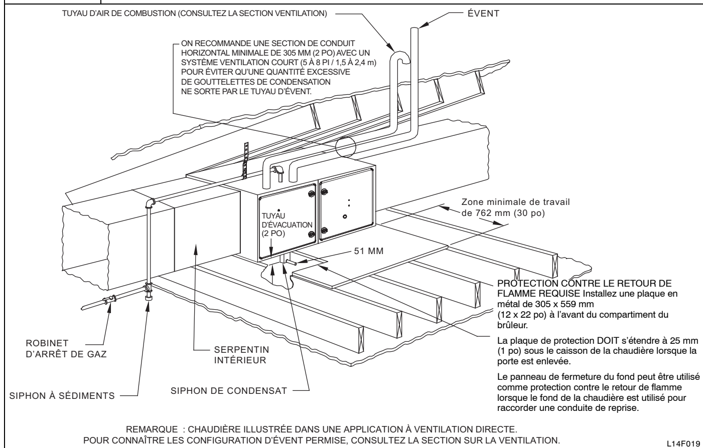
Figure 27 Plateforme de travail pour installation dans le grenier
