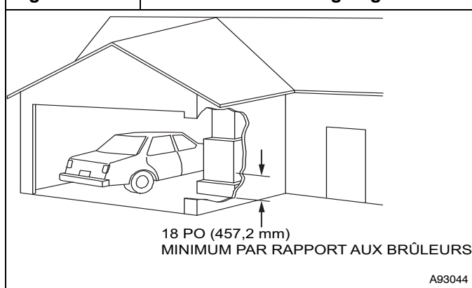
Figure 4 Installation dans un garage
