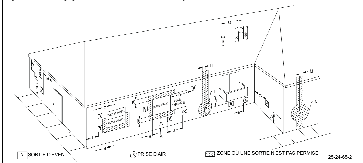
Figure 62 Dégagement des sorties d'évent d'un système à ventilation directe
