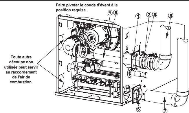
CONFIGURATION HORIZONTALE À GAUCHE ET VENTILATION À GAUCHE
