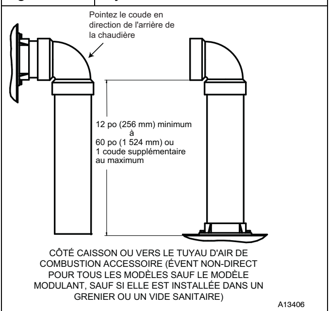
Figure 59 Tuyau d'air de combustion
