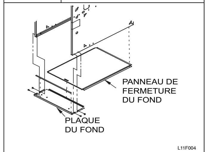
Figure 20 Retrait du panneau de fermeture du fond
