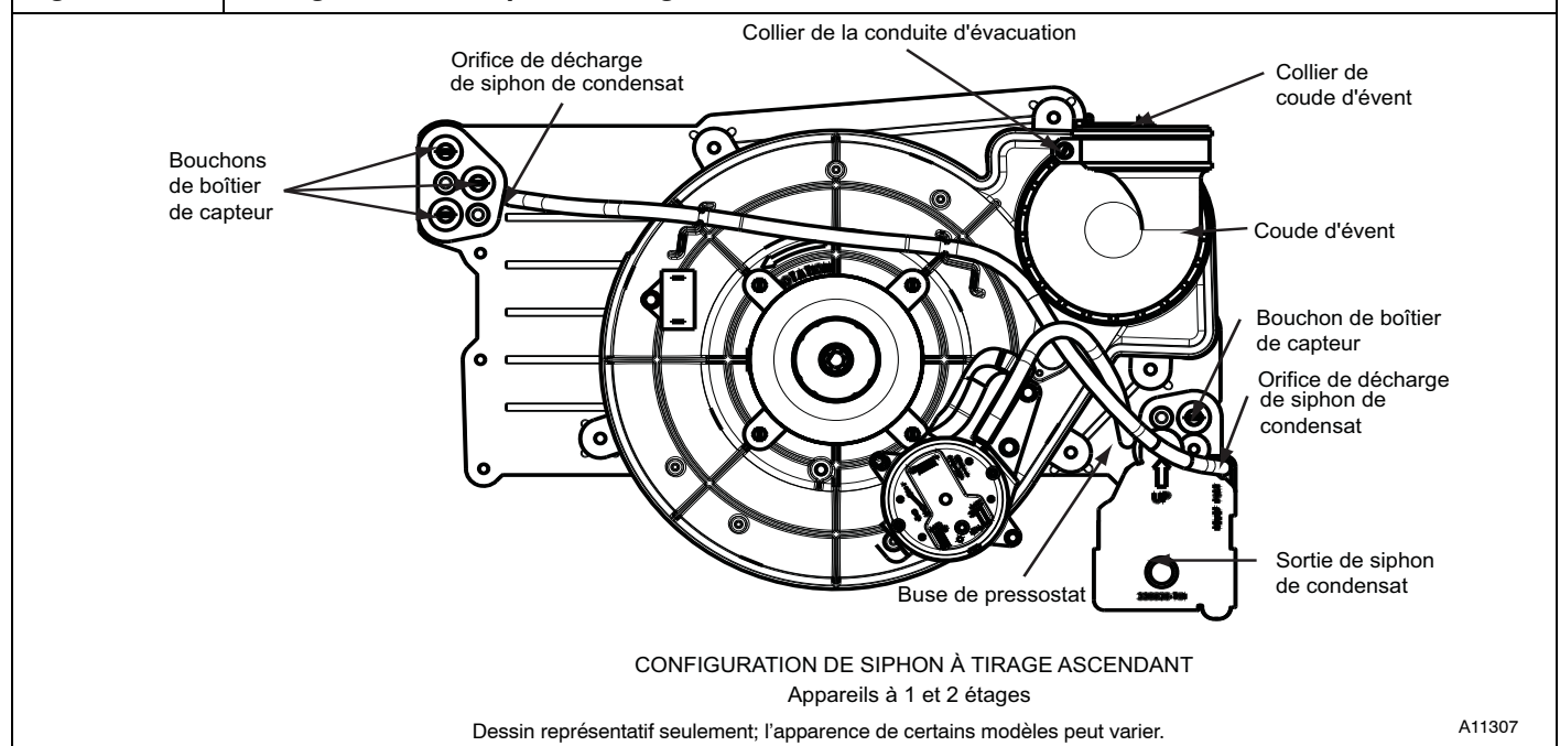
Figure 8 Configuration de siphon à tirage ascendant
