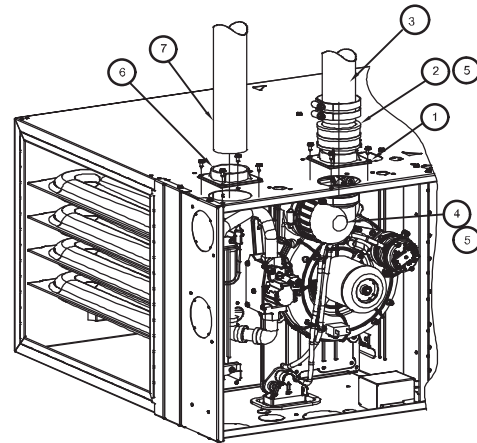
Figure 57 Configurations horizontales à gauche
