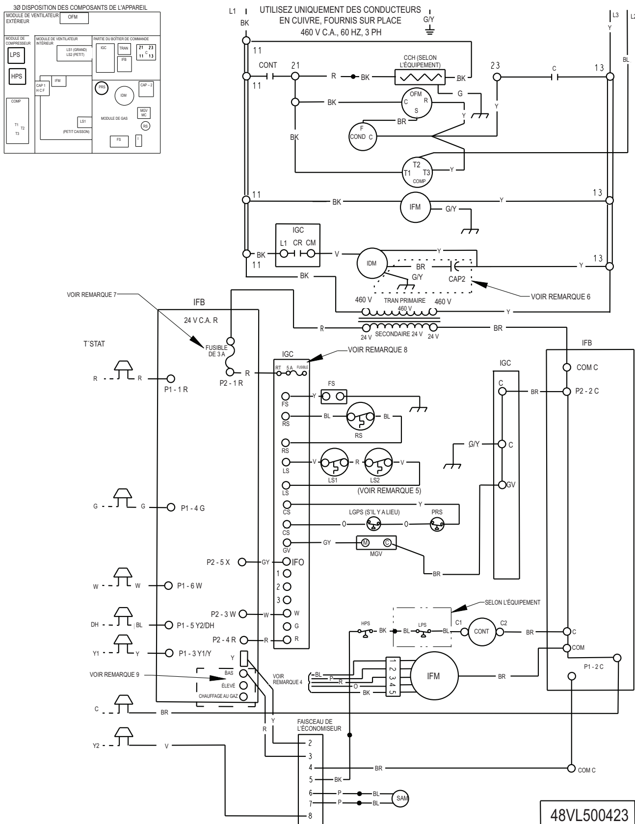
Figure 16, suite — Schéma de câblage en échelle — 460 V, 3 phases, 60 Hz
