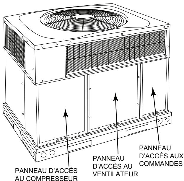
Figure 22 – Panneaux d'accès de l'appareil
