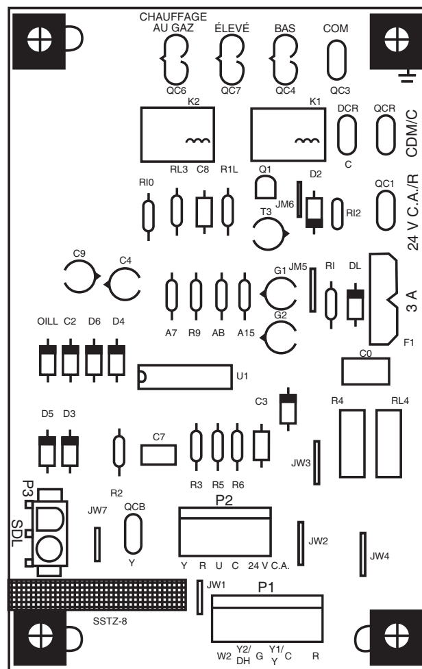
Figure 20 – Carte interface du ventilateur (IFB)
