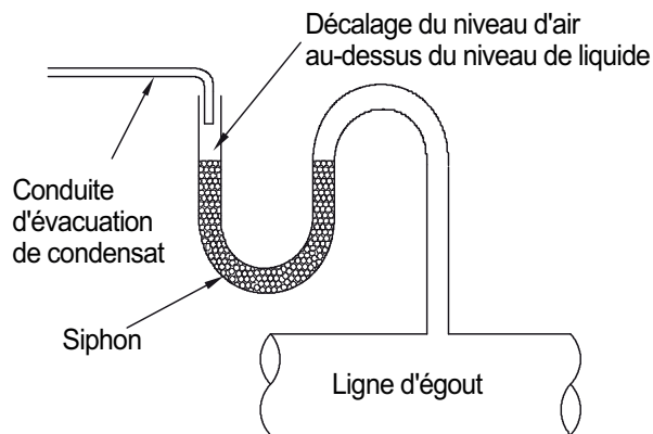
Figure 9 – Évacuation des condensats vers la conduite d'eaux usées
