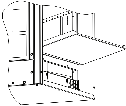
Figure 3 – Installation horizontale vers la droite de l'extension du bac (capacités 43, 60 et 61 seulement)
