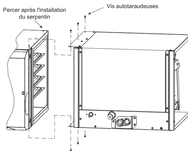
Figure 6 – Fixer le serpentin à l'appareil de chauffage
