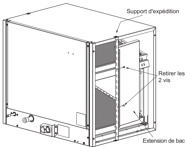
Figure 1 – Appareil de chauffage
