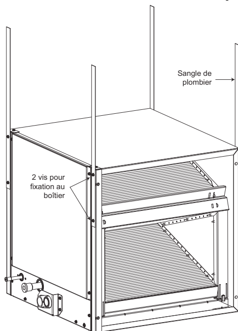
Figure 7 – Suspension du serpentin à l'aide de feuillard perforé
