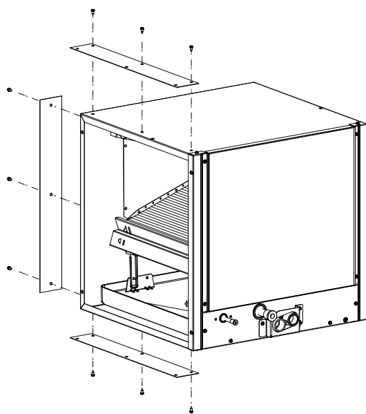
Figure 5 – Monter les plaques de fixation
