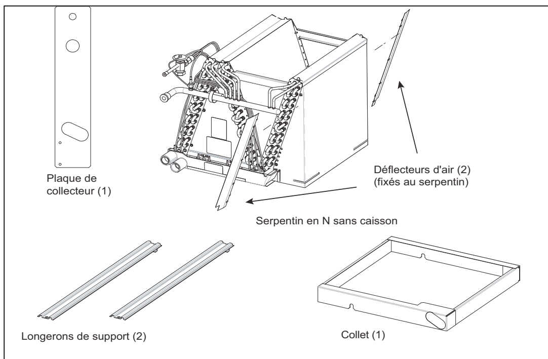
Figure 1 – Composants de serpentín en N sans caisson
