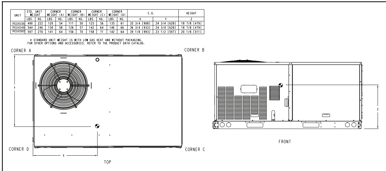
Fig. 2 - Dimensions
