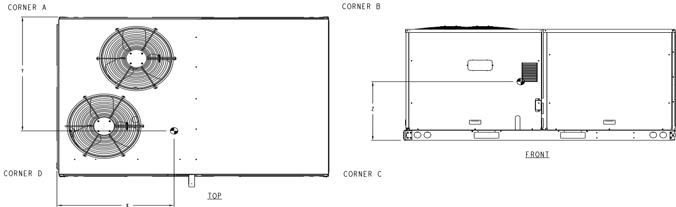
Fig. 6 – Dimensions RGH072 – 102
