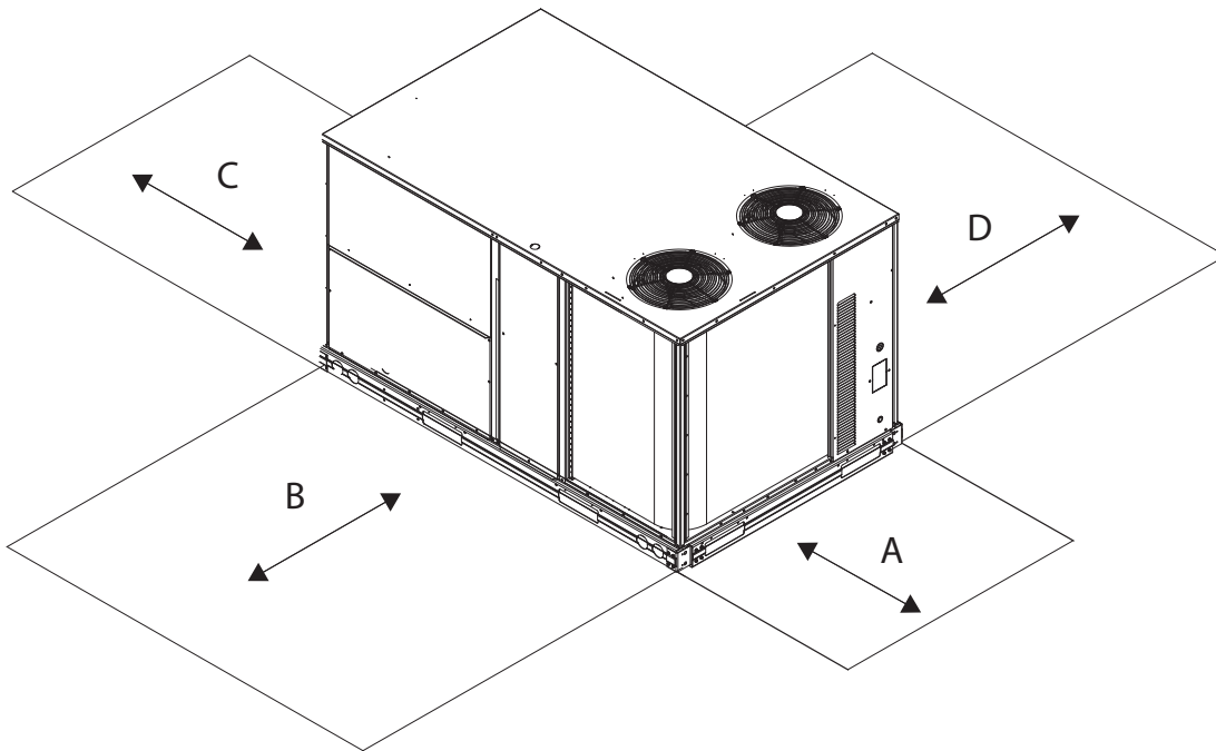
Fig. 6 – Dimensions RGH072 – 102
