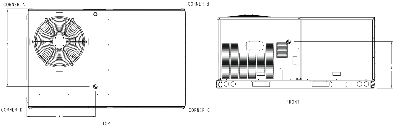
Fig. 2 - Dimensions RGH036-060
