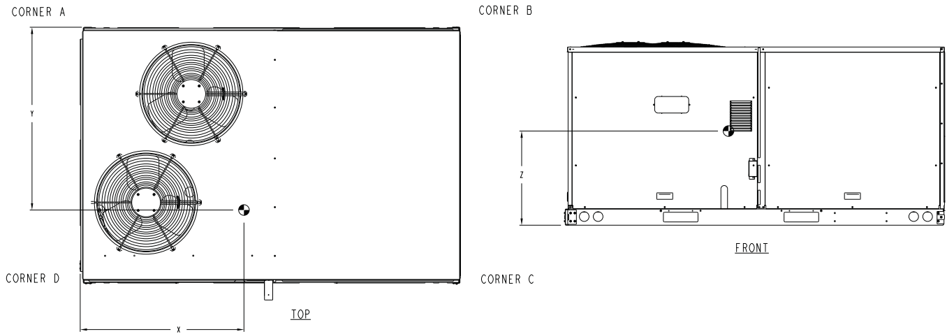
Fig. 6 - Dimensions RGH072 - 102
