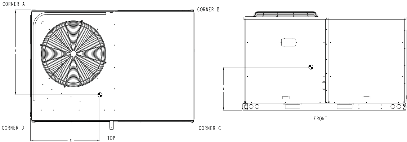
Fig. 9 - Dimensions RGH120
