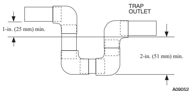
Fig. 7 - Condensate Trap
