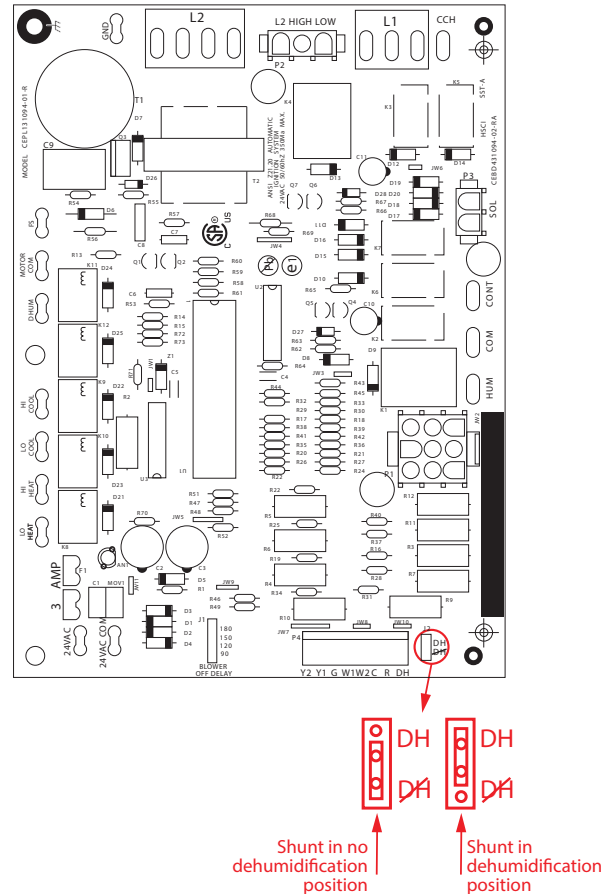
Fig. 17 - Interface Fan Board (IFB)
