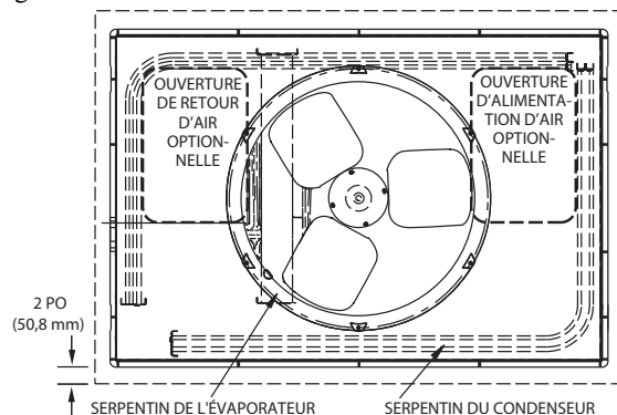
Figure 2 – Détails du montage sur dalle
