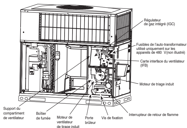
Figure 18 – Compartiment de ventilateur et boîtier de fumée
