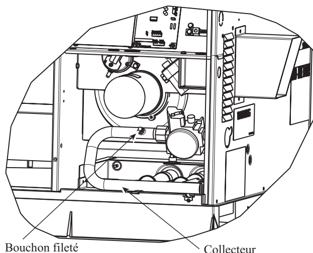
Figure 11 – Ensemble de brûleur
