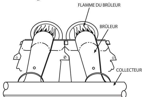
Figure 12 – Brûleur monoport
