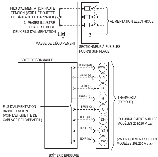
Figure 10 – Branchements haute et basse tensions
