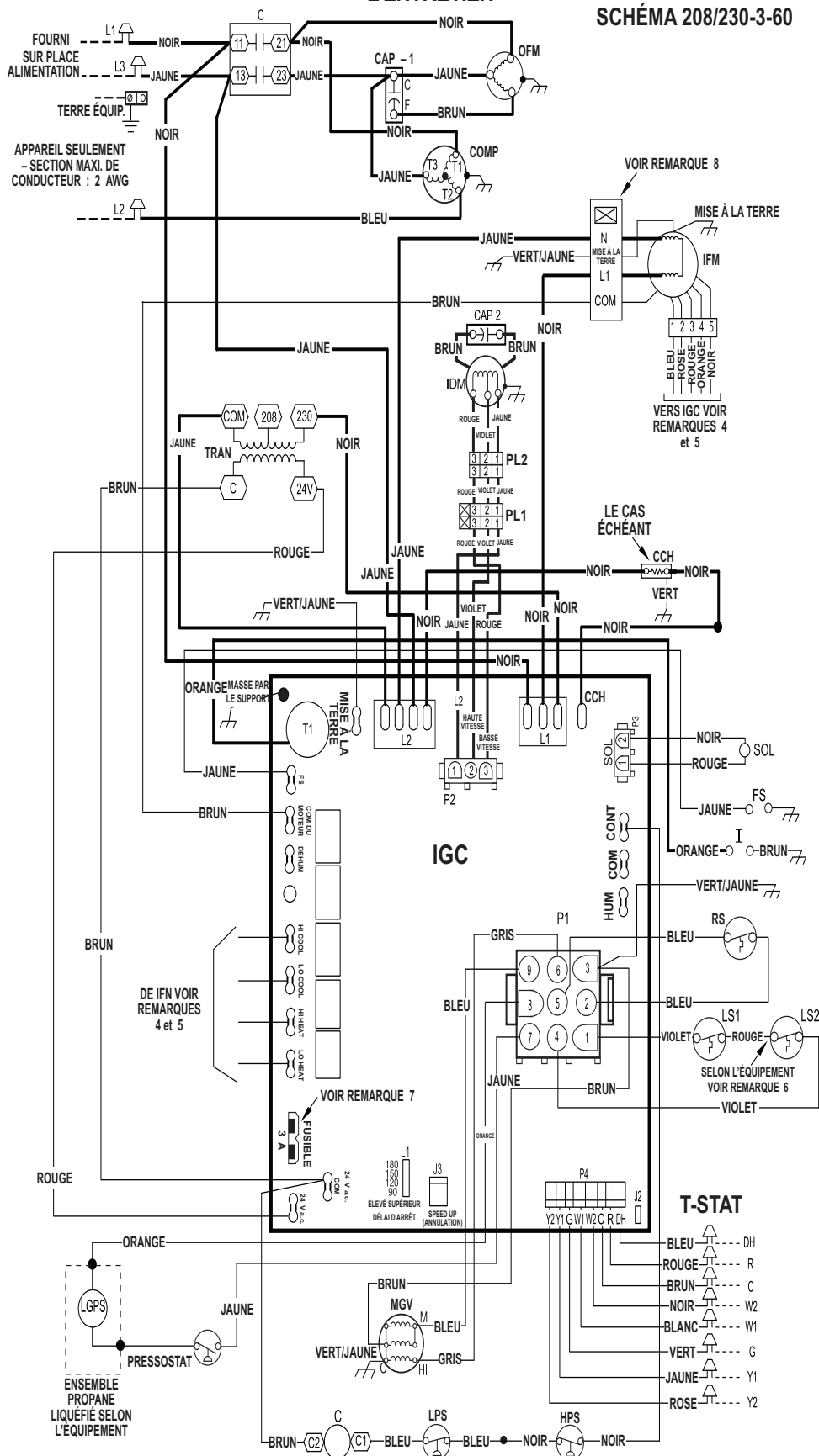
Figure 15 – Modèles 208/230 V 3 phases 60 Hz Schéma de connexion de câblage, pouvoirs calorifiques 40, 60 et 90 KBtu/h
