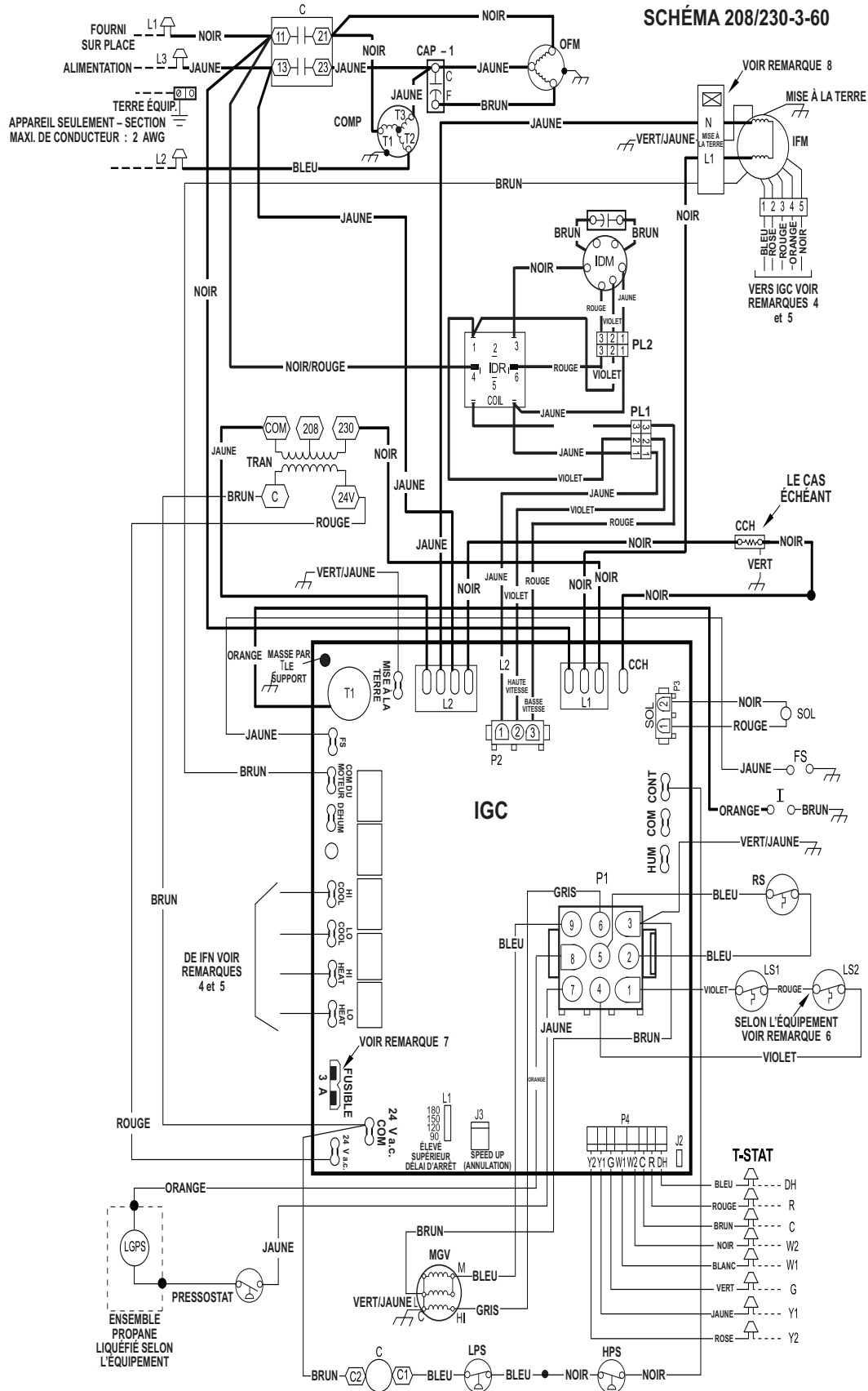
Figure 16 – Modèles 208/230 V 3 phases 60 Hz Schéma de connexion de câblage, pouvoirs calorifiques 115 et 130
