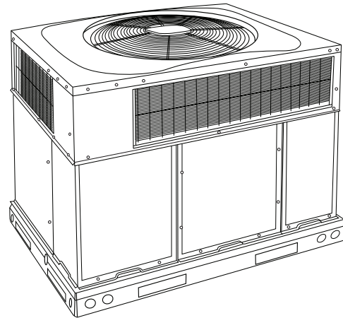
Figure 1 – Appareil PGR5 (modèle à faible concentration de NOx disponible)
