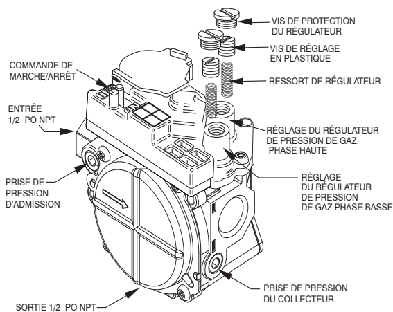
Figure 13 – Vanne de gaz à deux étages
