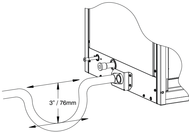
Fig. 8 - Condensate Trap
