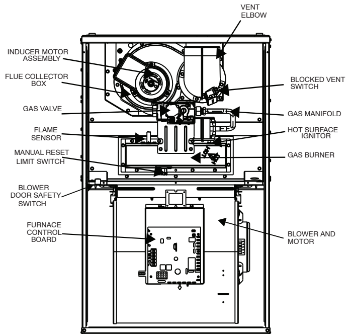
Fig. 1 – 80% AFUE Single Stage Furnace Components A180221
