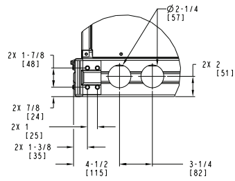
DETAIL B TYP 2 PLCS
