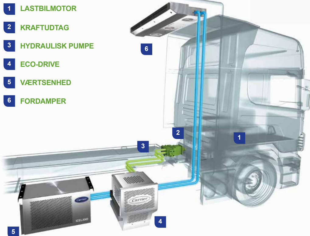
LASTBIL- MOTOR
