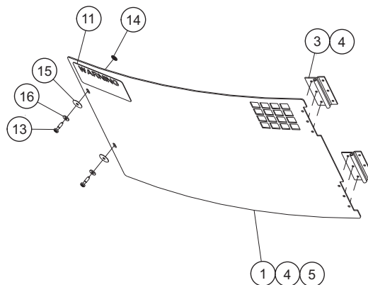
Door Assembly
